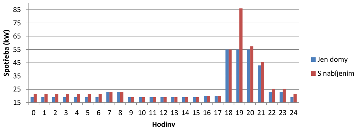
Graf 14: Spotřeba 10 domů s 5 auty nabíjenými přes noc a 5 v jednu hodinu v zimě
