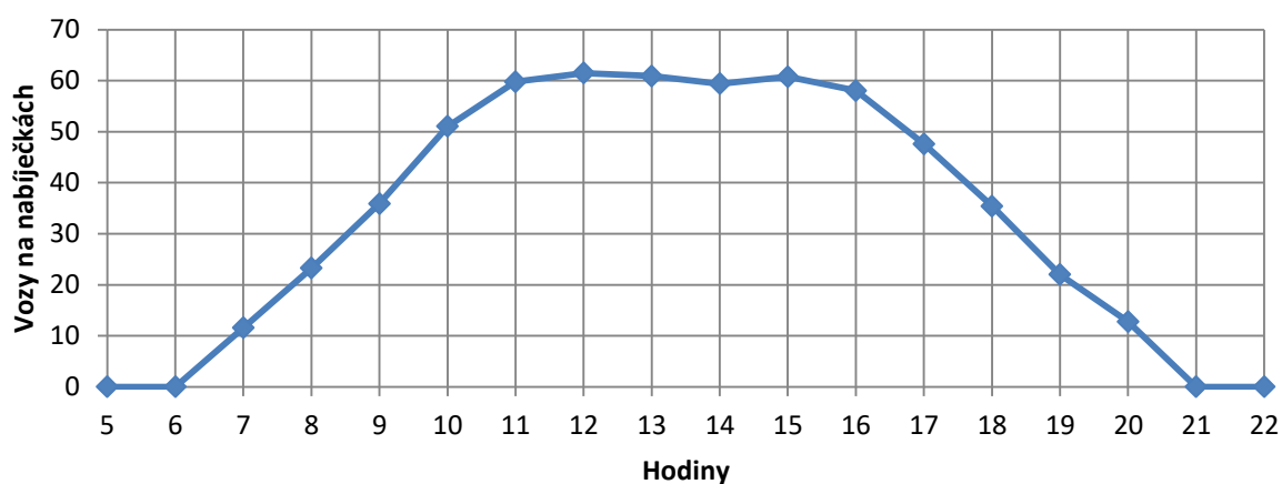
Graf 21: Vytíženost nabíječek s 12,3% elektromobilů o víkendu
