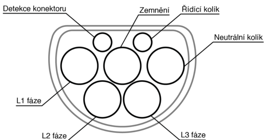
obr. 2-25 Konektor Mennekes
