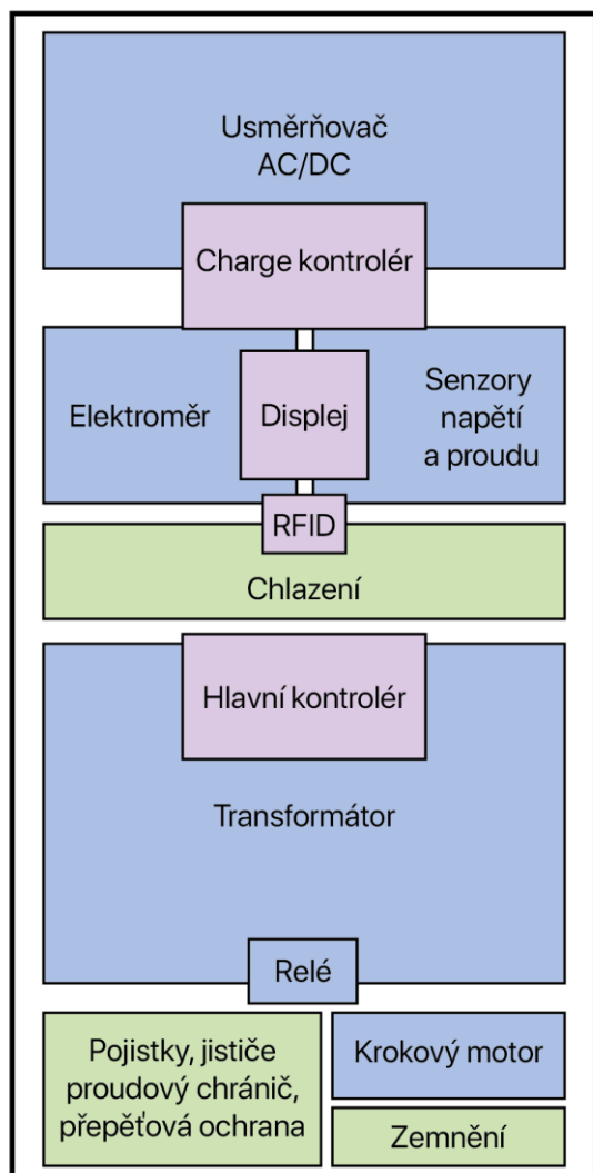
obr. 2-22 Vnitřní schéma ucelené rychlé dobíjecí stanice
