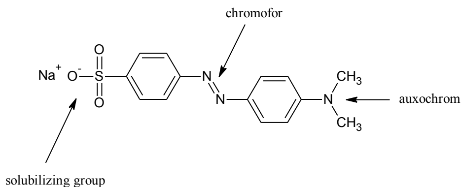
Obr. 6: Rozdělení přítomných skupin v barvivu methyloranž [31]
