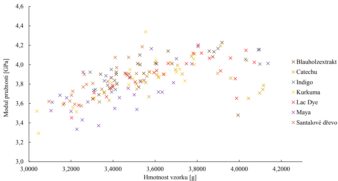
Obr. 55: Závislost naměřených hodnot modulu pružnosti v ohybu na hmotnosti vzorku
