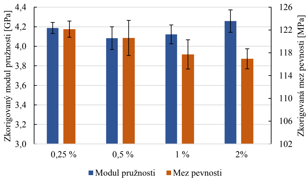
Obr. 63: Zkorigované hodnoty měřených mechanických vlastností v ohybu pro různé koncentrace bio-barviva Santalové dřevo
