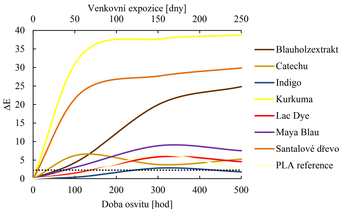
Obr. 31: Závislost \Delta E na době osvitů
