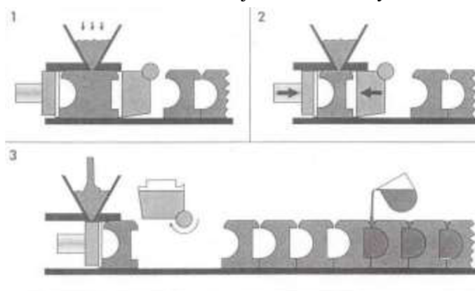
Obr. 6 Výroba forem a odlitků na lince DISA [17]
