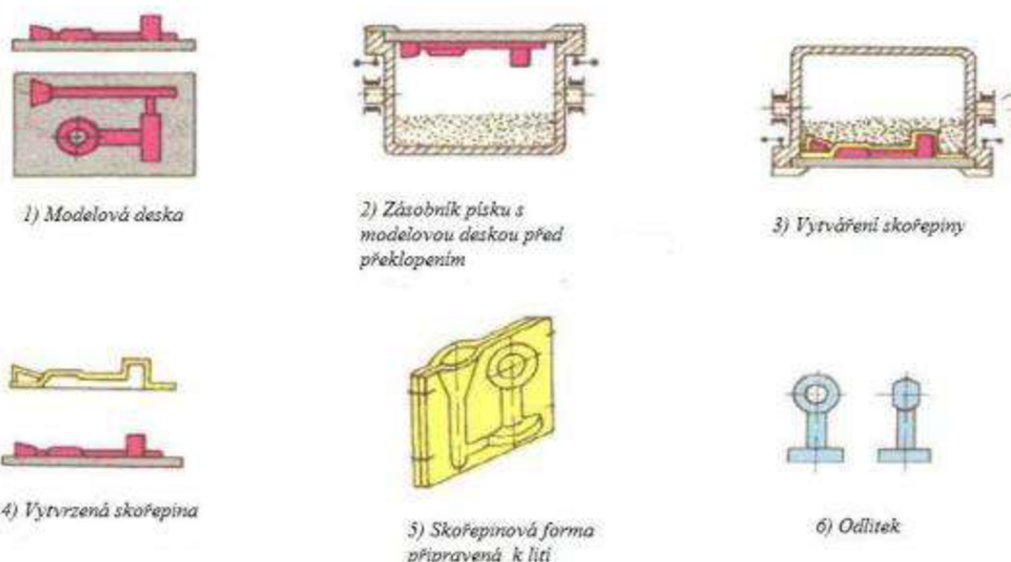
Obr. 3 Postup při výrobě formy metodou C [10]
