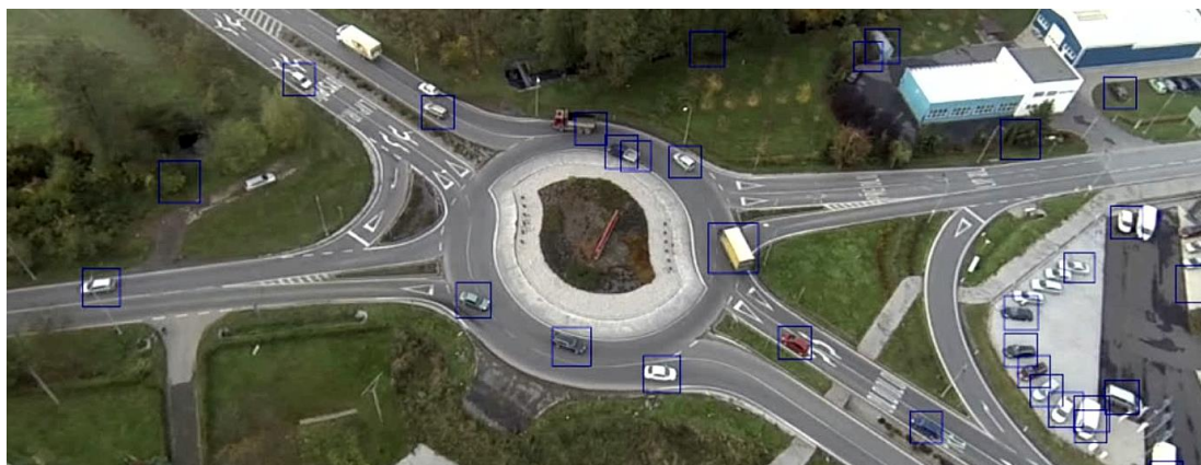
Obr. 3 Výsledek práce klasifikátorů při detekci vozidel
