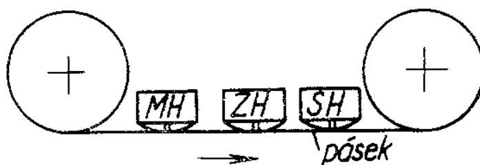
(obr. 7: Schéma magnetofonu; MH = mazací hlava, ZH = záznamová hlava, SH = snímací hlava)
