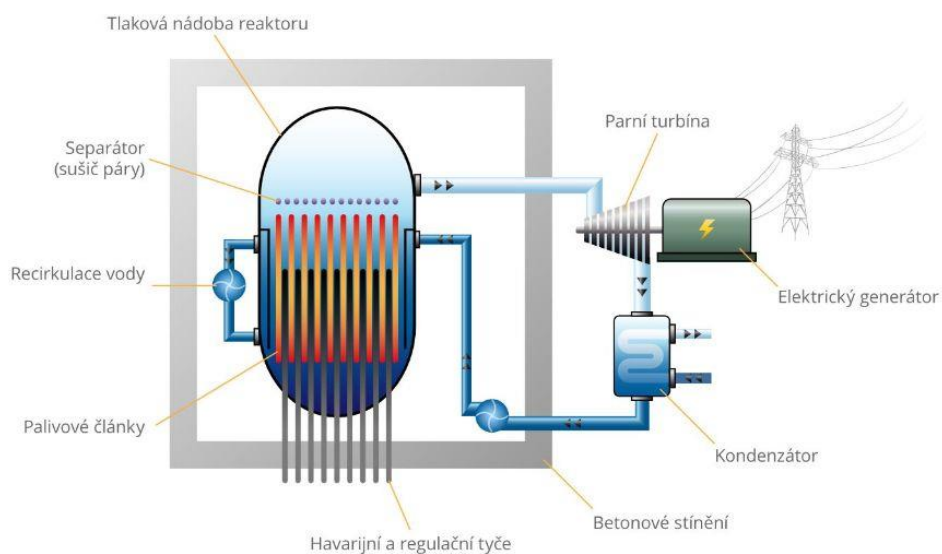
Obrázek 2 Varný reaktor (Základní typy jaderných reaktorů, 2019)
