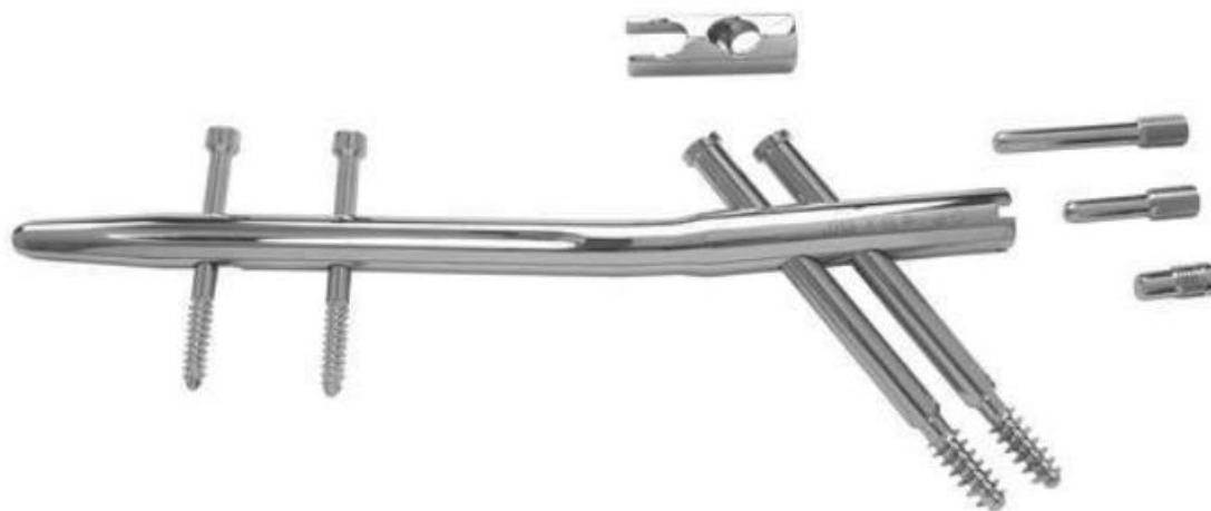
Obrázek 15 Krátký rekonstrukční hřeb
