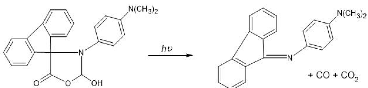
Obrázek 14 Odštěpení anhydridu a vznik iminu. Dozimetr se zbarví do červena. 32
