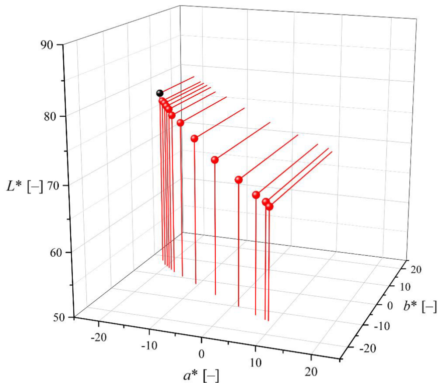
Obrázek 32 Znáznornění barevné změny v barvovém prostoru L^*a^*b^* pro vzorek nanosený Bakerovým pravítkem 60. Počáteční bod je vyznačen černě
