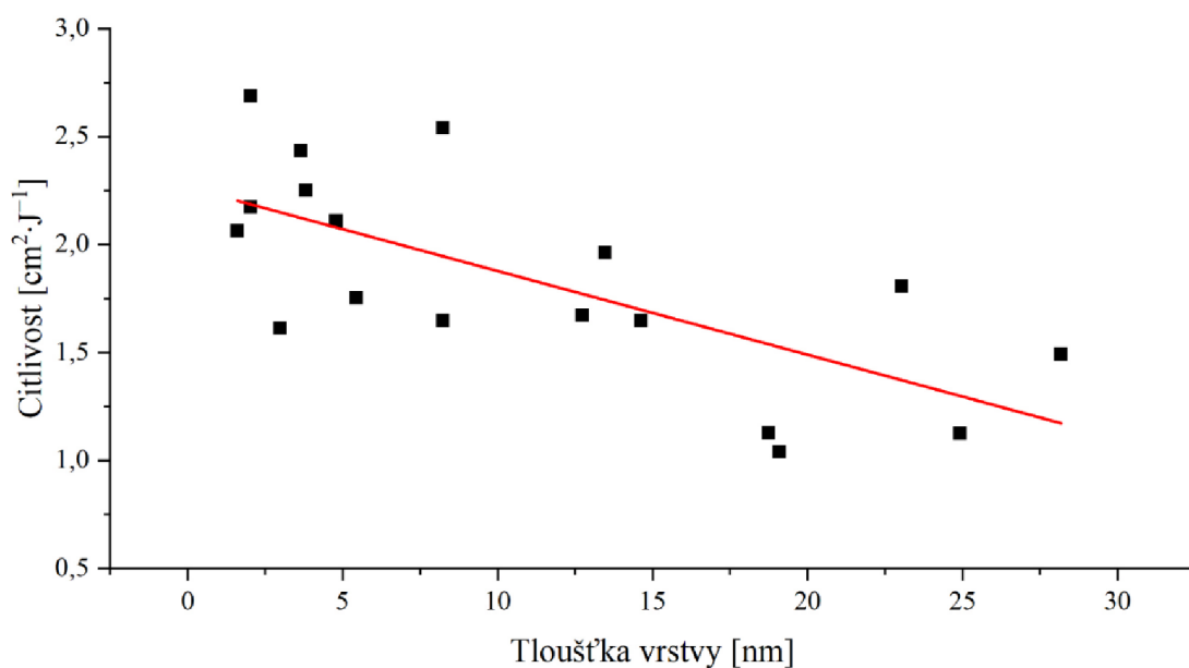
Obrázek 34 Závislost citlivosti na tloušťce vrstvy. Citlivost byla vypočítána z průměrné dávky ozáření dle \sigma^* = 0 pro danou nanášecí techniku. Obdobně i tloušťka vrstvy je průměrem pro danou nanášecí techniku.
