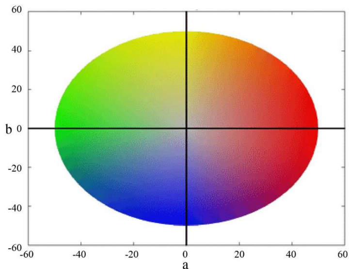
Obrázek 31 Znáznornění změny barev v barvovém prostoru L^*a^*b^* při měrné světlosti L^* = 50 cit. 45
