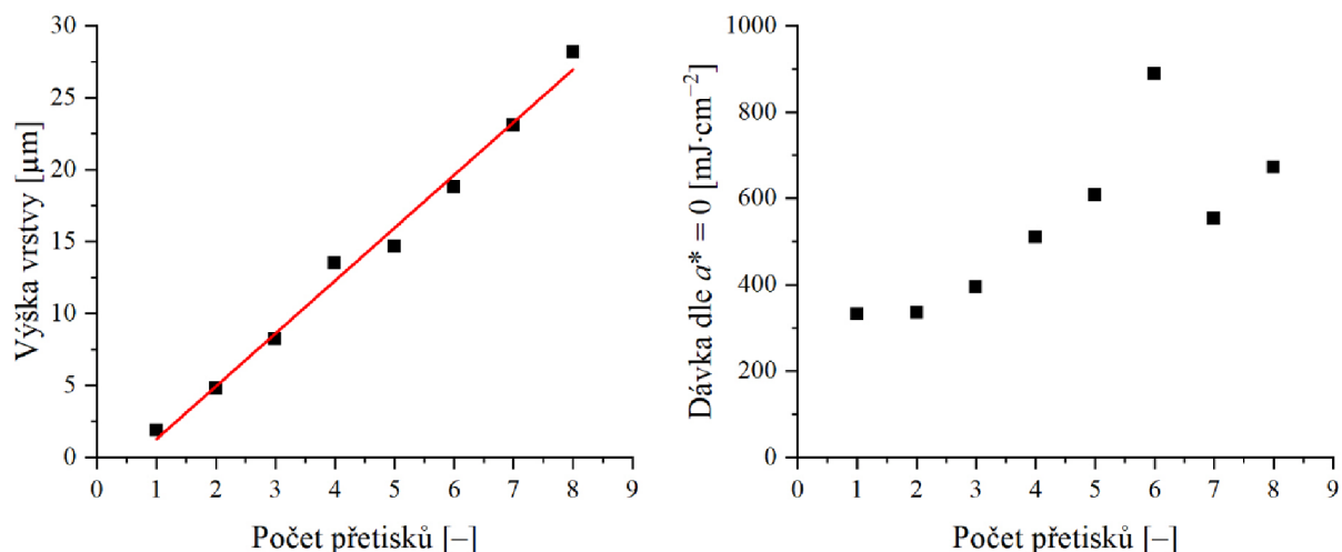
Obrázek 33 Závislost výšky vrstvy a dávky ozáření dle \sigma^* = 0 na počtu přetisků u kompozic ze stejné série
