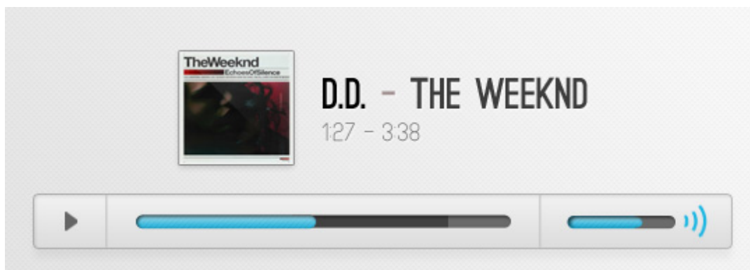
Obr. 2.4: Prehrávač jPlayer
