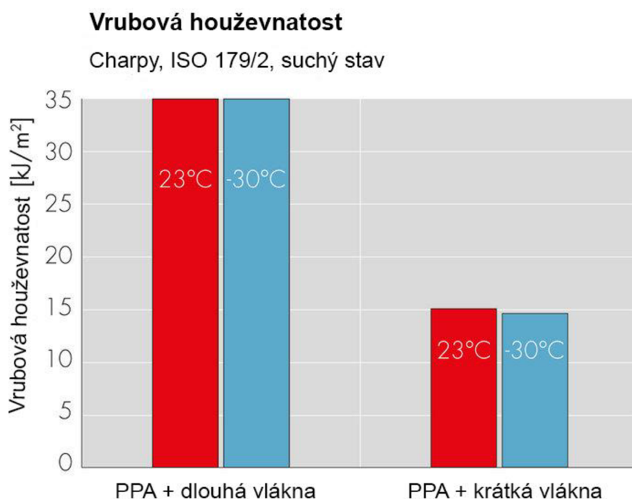
Obr. 2.5 Porovnání vrubové houževnatosti dvou materiálů se stejnou matricí, vlevo vyztuženého pomocí dlouhých vláken, vpravo vlákny krátkými [15]
