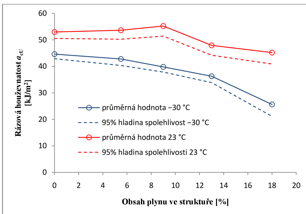
Obr. 3.15 Porovnání průběhů rázové houževnatosti v závislosti na obsahu plynu v polymeru při teplotách +23 °C a -30 °C
