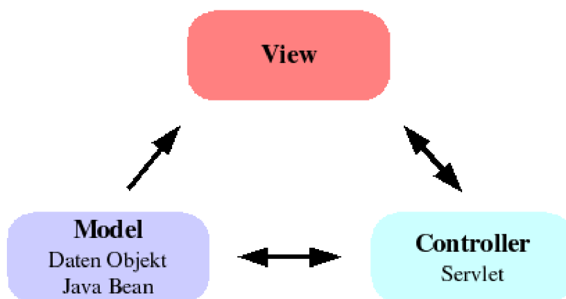
Obrázek 2.1. Princip architektury MVC. Převzato z [1].
