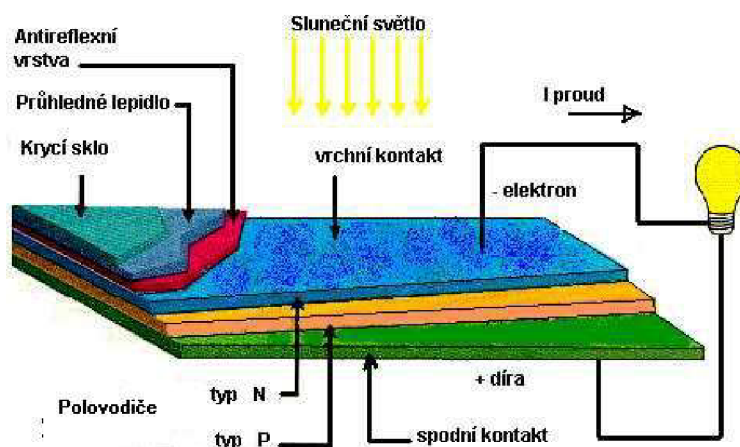
Obrázek 14 Fotovoltaický článek [49]
