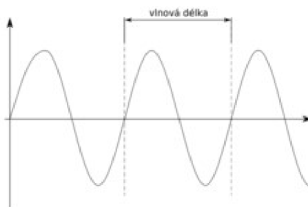
Obrázek 4 Vlnová délka [13]
