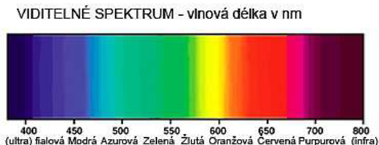
Obrázek 9 Viditelné spektrum [18]
