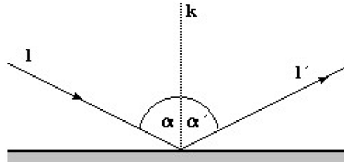
Obrázek 5 Odraz vlnění [46]
