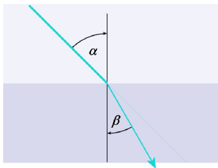
Obrázek 6 Lom vlnění [47]
