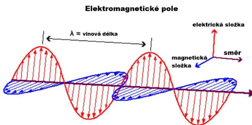
Obrázek 3 Elektromagnetické pole [34]
