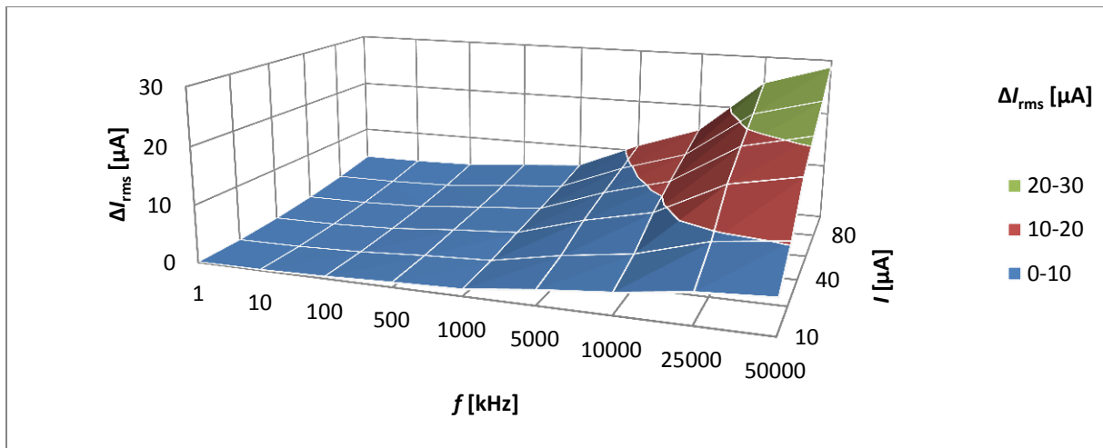
Obrázek 58: Závislost absolutní chyby \Delta I_{rms} na frekvenci f a proudu I pro tranzistor T_{11} W/L = 10/10 \mu\text{m}
