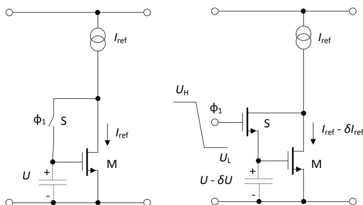
Obrázek 9: Proudová paměťová buňka druhé generace: (a) s ideálním spínačem, (b) s MOS spínačem [10]
