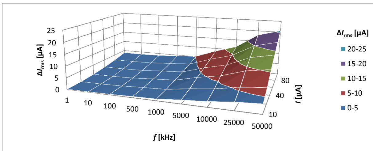
Obrázek 59: Závislost absolutní chyby \Delta I_{rms} na frekvenci f a proudu I pro tranzistor T_{11} W/L = 1/0,7 \mu\text{m}
