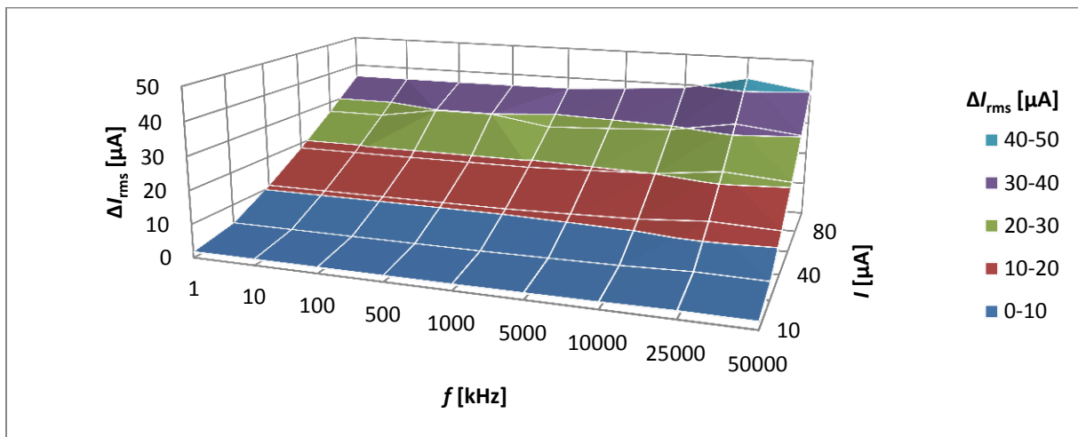
Obrázek 27: Závislost absolutní chyby \Delta I_{rms} na frekvenci f a proudu I pro tranzistor W/L = 1/0,7 \mu m
