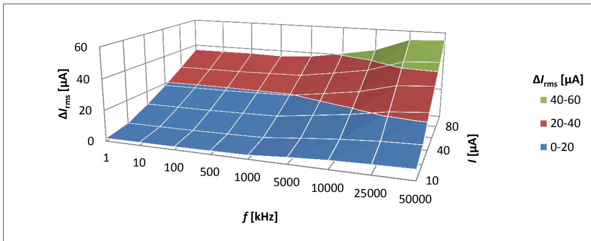
Obrázek 26: Závislost absolutní chyby \Delta I_{rms} na frekvenci f a proudu I pro tranzistor W/L = 10/10 \mu m
