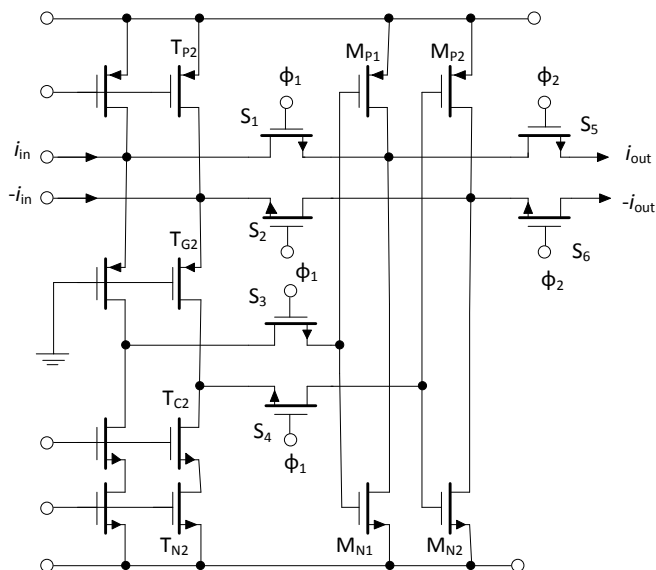
Obrázek 3: Plně diferenční paměťová buňka třídy AB [6]
