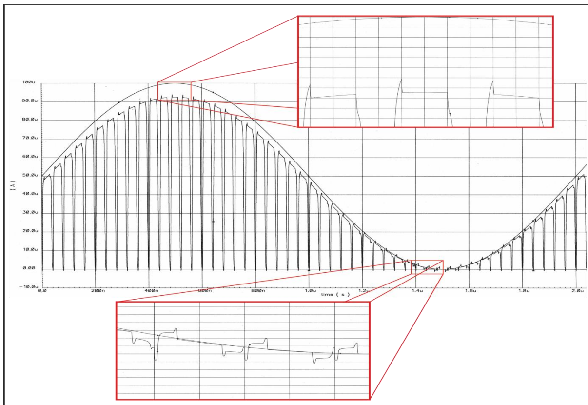
Obrázek 66: Časový průběh pro NMOS Dummy spínač o rozměrech W/L = 1/1 \mu\text{m} a Dummy W/L = 0,5/1 \mu\text{m}
