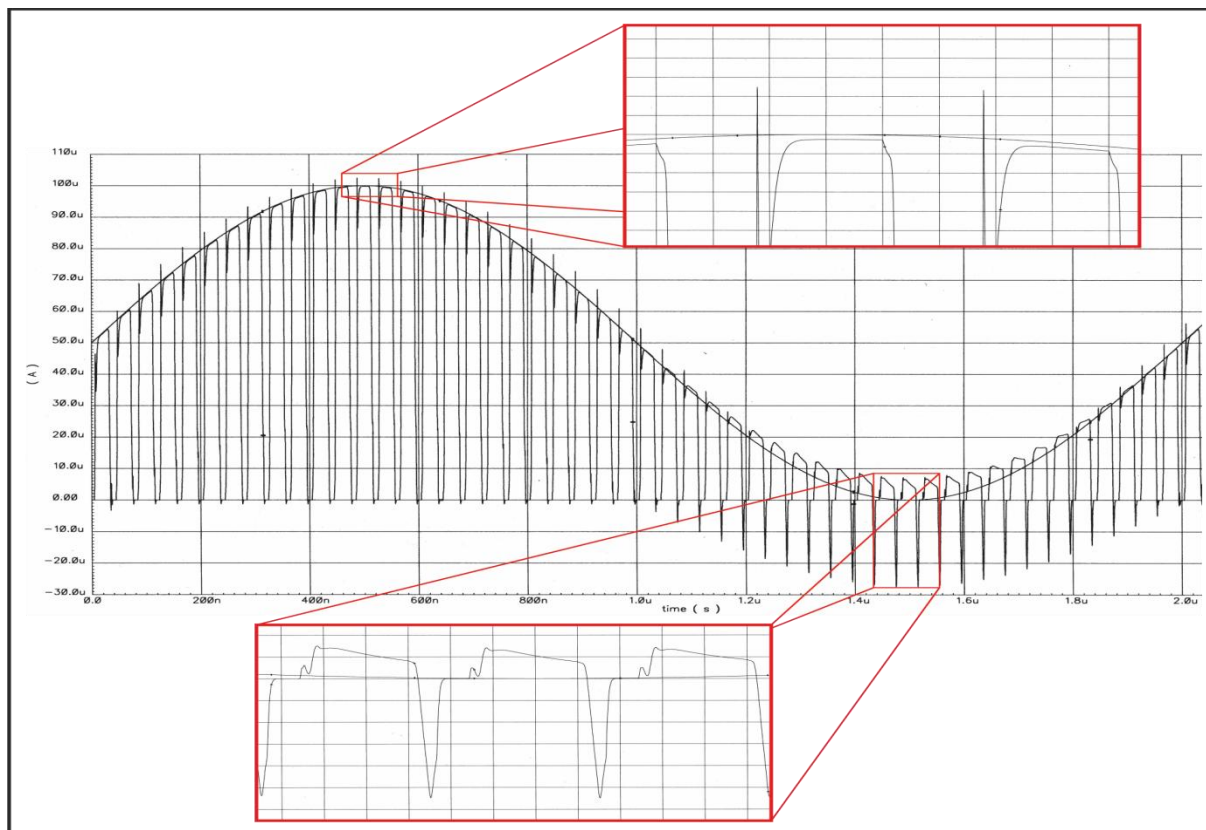
Obrázek 68: Časový průběh pro Bootstrapped spínač o rozměrech spínacího tranzistoru NMOS T_{11} W/L = 20/0,7 \mu\text{m} , ostatních tranzistorů W/L = 1/0,7 \mu\text{m} a velikosti kondenzátorů C_1 až C_3 = 1 \text{ pF}
