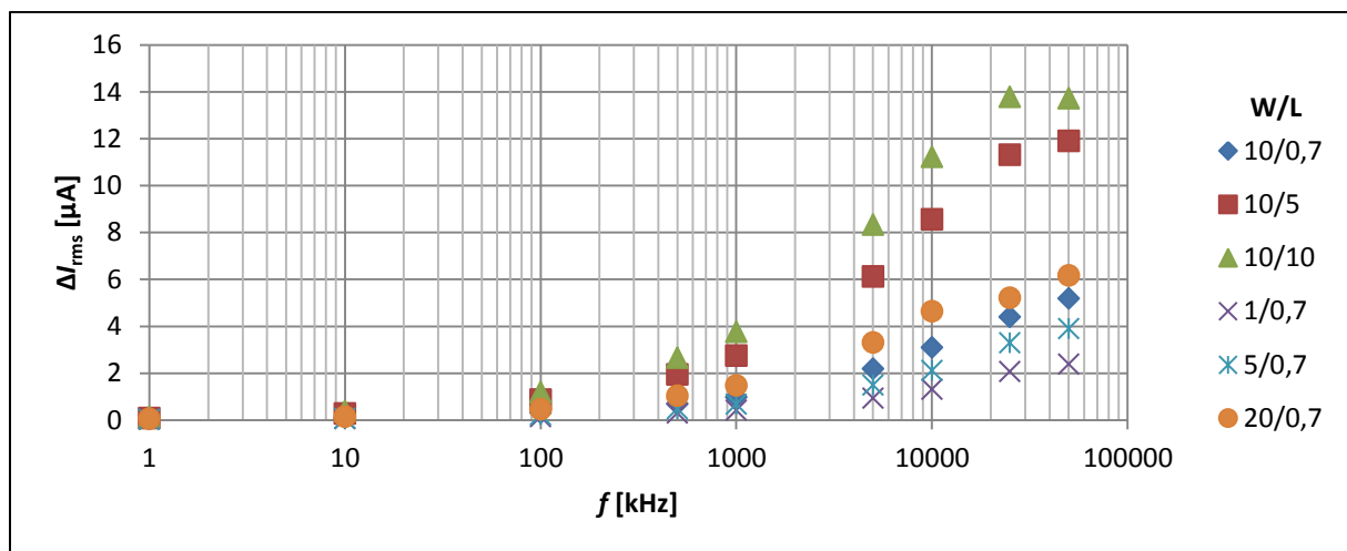
Obrázek 16: Závislost absolutní chyby \Delta I_{rms} na frekvenci f a rozměrech tranzistoru W/L pro vstupní proud I = 10 \mu\text{A}
