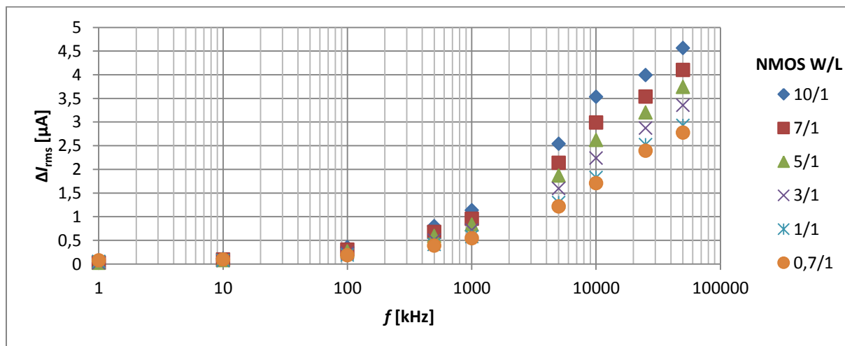
Obrázek 31: Závislost absolutní chyby \Delta I_{rms} na frekvenci f a rozměrech NMOS tranzistoru W/L k antiparalelně připojenému PMOS tranzistoru W/L = 10/1 μm pro vstupní proud I = 10 \mu A
