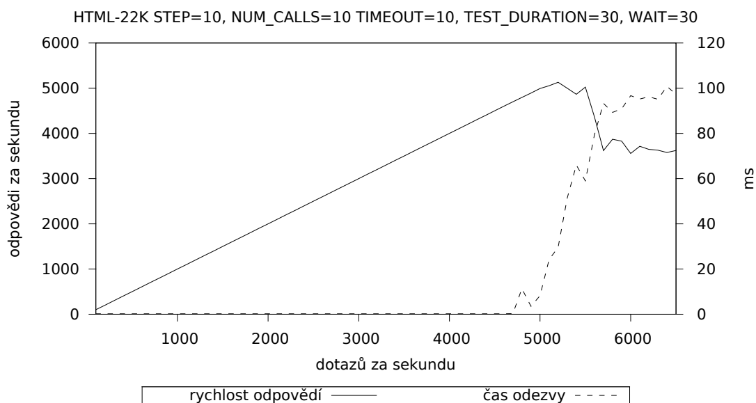
Obrázek 6.1: Graf výsledku testování na statický html soubor o velikosti 12 KiB
