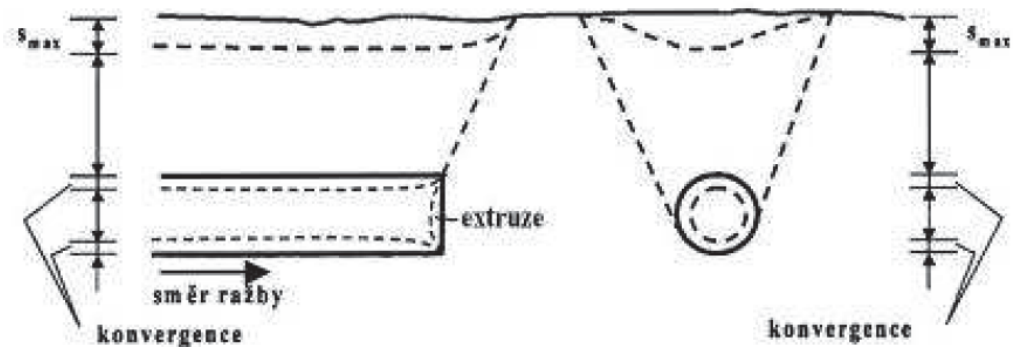
Obr. 7: Tvar poklesové kotliny v důsledku ražby
