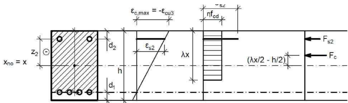
Obr. 32: Namáhání průřezu v bodě 1
