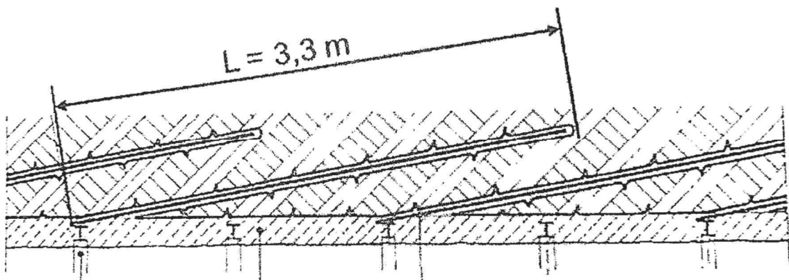
Obr. 6: Zajištění výrubu pomocí jehel a stříkaného betonu, Westtangent Bochum [1],
