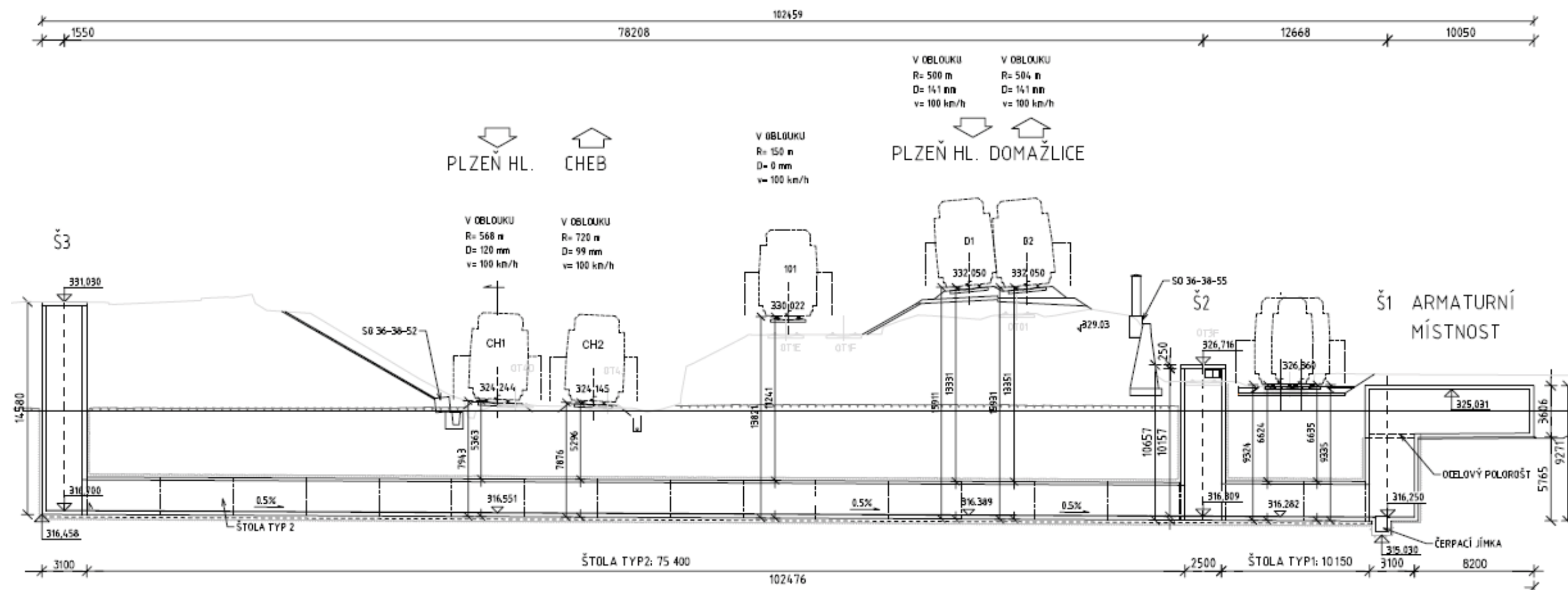
Obr. 3: Podélný řez kolektorem [ 4]
