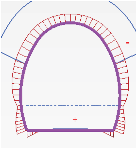
řez 1, fáze 5: N_{max} = -11,4 \text{ kN/m} N_{min} = -172,2 \text{ kN/m}
