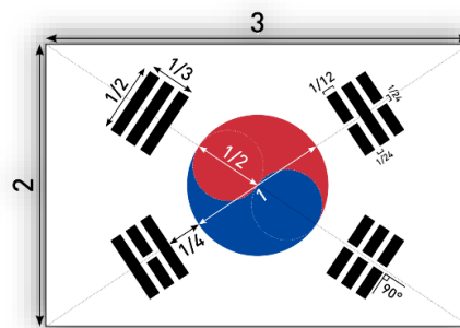
Obrázek 6: parametry vlajky
