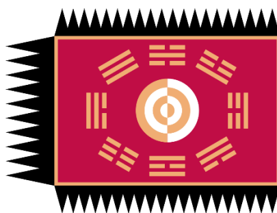
Obrázek 2: čosonská standarda
