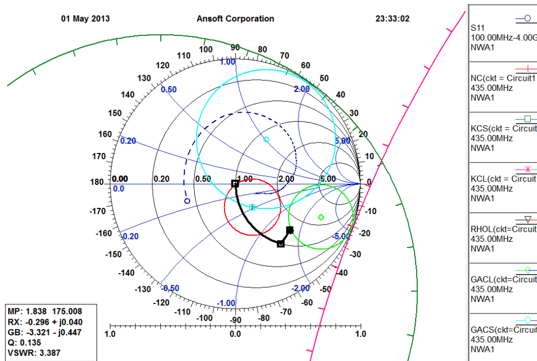
Obr. 2.9: Výkonové přizpůsobení
