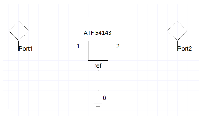
Obr. 2.4: Schéma pro vyšetření stability
