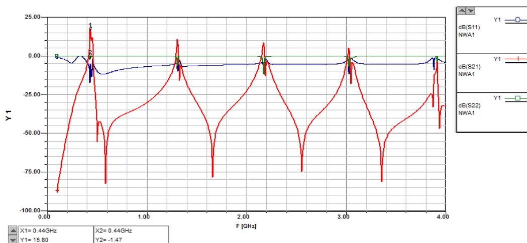
Obr. 2.17: Širokopásmová analýza filtru
