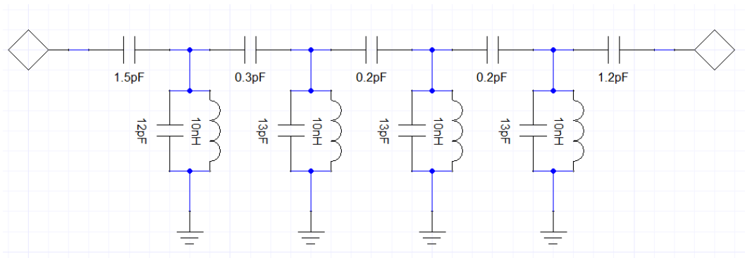
Obr. 2.12: Schéma filtru s reálnými hodnotami součástek
