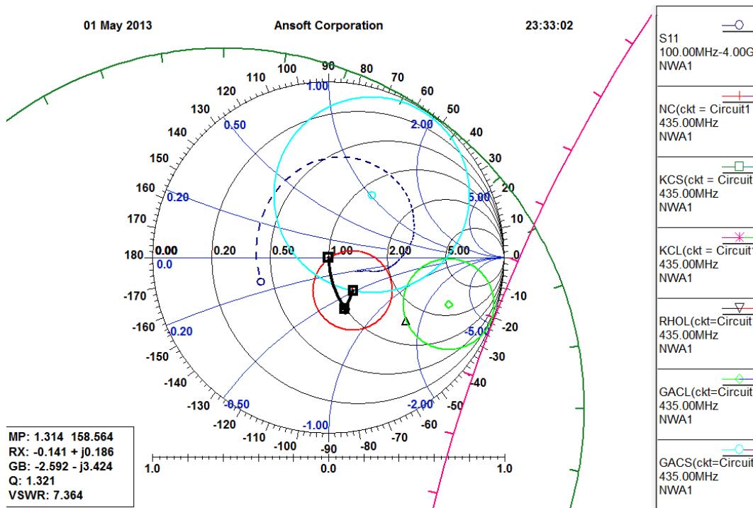
Obr. 2.8: Šumové přizpůsobení
