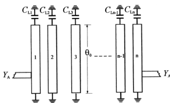
Obr. 1.4: Základní konfigurace kombinovaného filtru[4]
