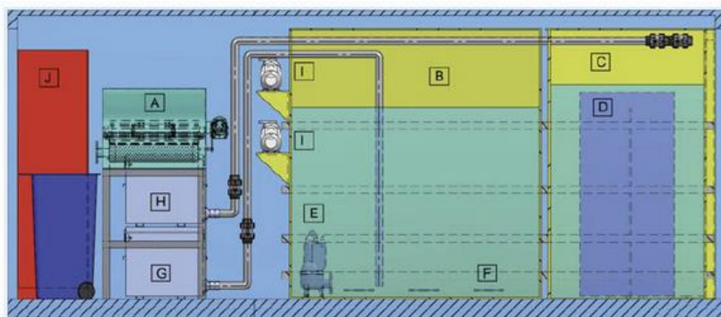
Obr. č. 6.3 - Zjednodušené funkční schéma ČOV AS-ISO MBR (Asio.cz)
