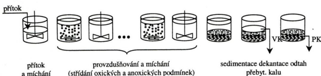
Obr. č. 3.5 – Schéma SBR procesu (Hlavínek a kol. 2003)
