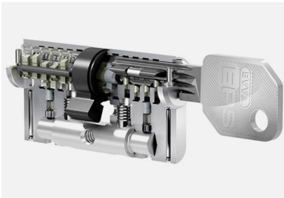
Obrázek 14: Bezpečnostní vložka s klíčem (Zdroj: [18])
