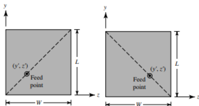
Obrázek 1.6 Kruhově polarizovaná téměř čtvercová flíčková vlevo LHCP, vpravo RHCP [1]
