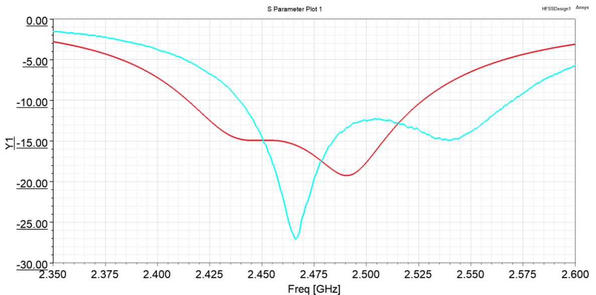
Obrázek 3.3 Zobrazovaný frekvenční posun u antény bez inkluze u středního vodiče, červená – simulace, modrá - měření
