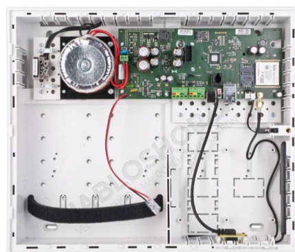
Obrázek 4.1: Ústředna JA-106K [10]
