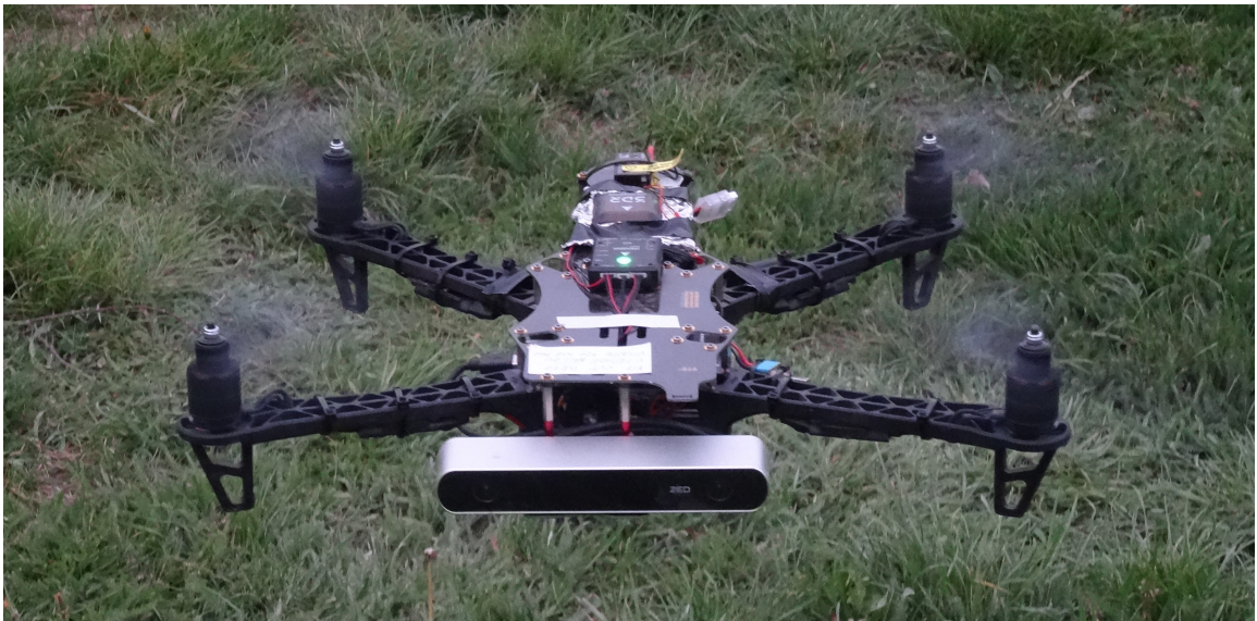
Obrázek 5.1: Testovací dron s řídicí jednotkou Pixhawk, stereoskopickou kamerou ZED a superpočítačem Nvidia Jetson vyfocený za letu těsně nad zemí.
