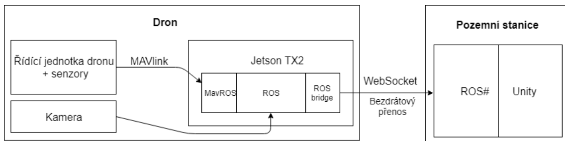
Obrázek 3.6: Komunikační protokoly mezi dronem a aplikací. Na straně aplikace zprostředkovává komunikaci knihovna ROS#, která komunikuje s dronem přes ROSbridge, který je přenášející přes protokol WebSocket.
