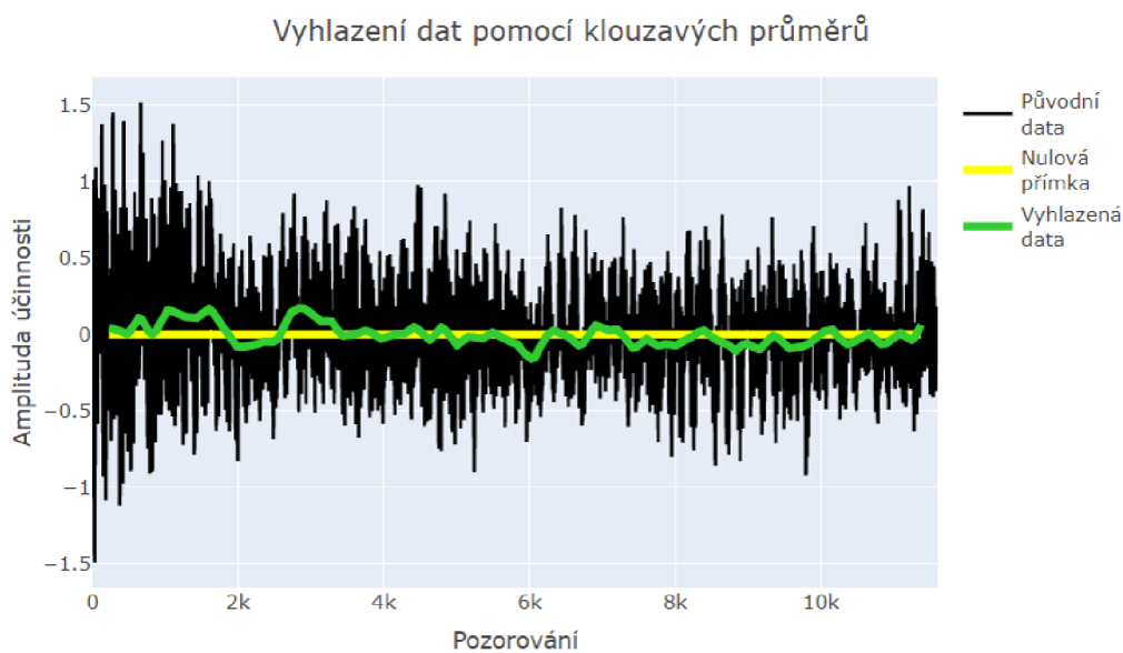
Obrázek 12: Vyhlazení dat4a pomocí klouzavých průměrů
