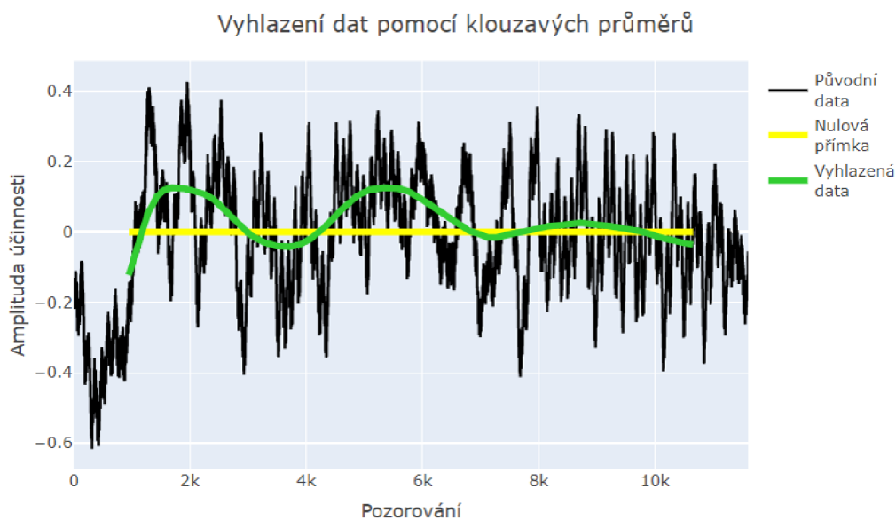
Obrázek 19: Vyhlazení dat 2c pomocí klouzavých průměrů
