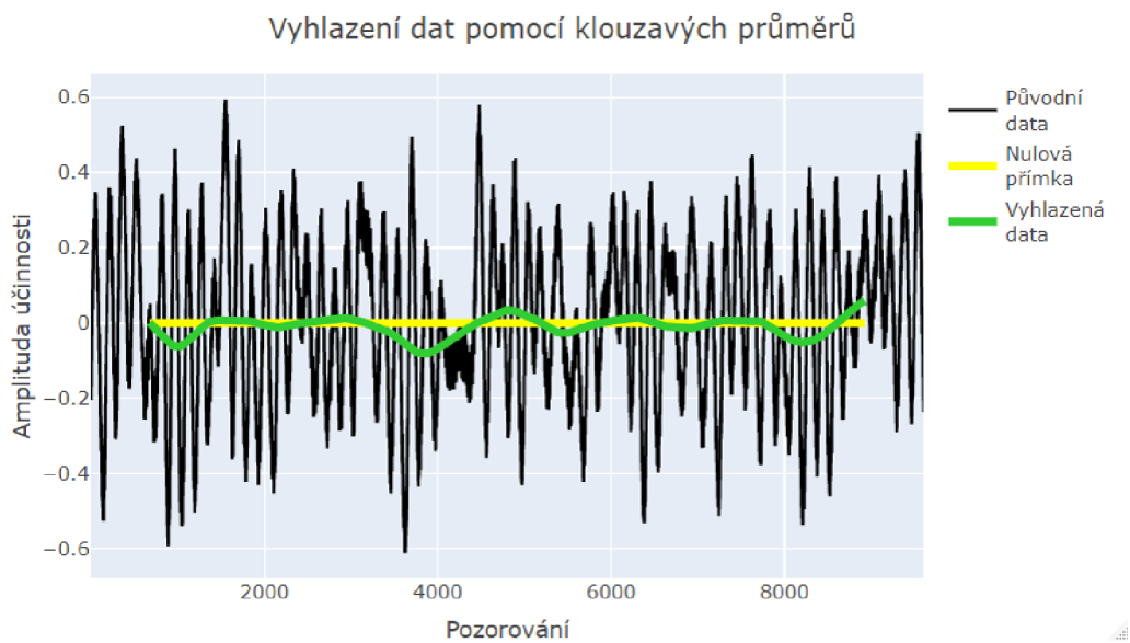
Obrázek 15: Vyhazení dat1b bez prvních 2000 pozorování pomocí klouzavých průměrů
