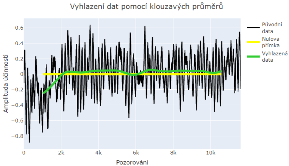
Obrázek 14: Vyhazení dat1b pomocí klouzavých průměrů
