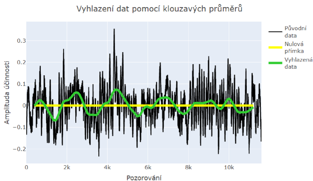
Obrázek 17: Vyhlazení dat3c pomocí klouzavých průměrů
