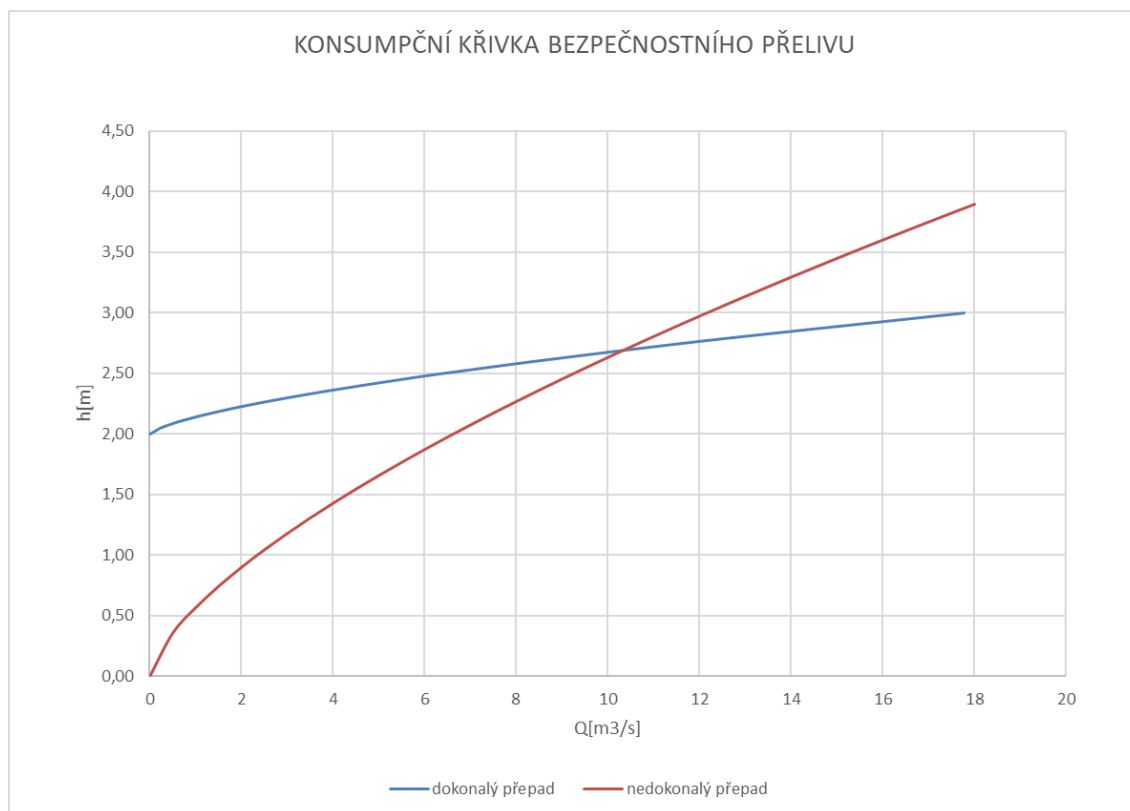
Graf 3: Konzumpční křivka bezpečnostního přelivu
