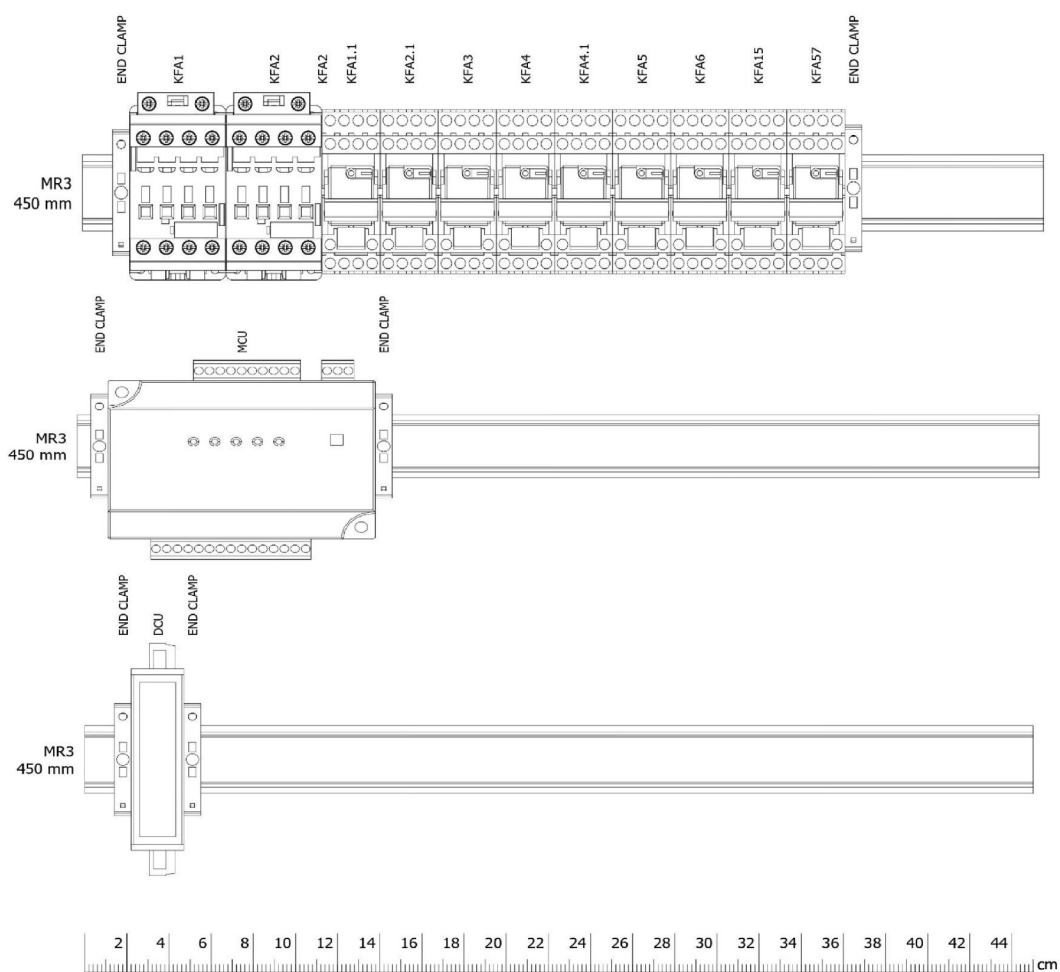
Obr. 6.1: Porovnanie radiacích častí zapojení
