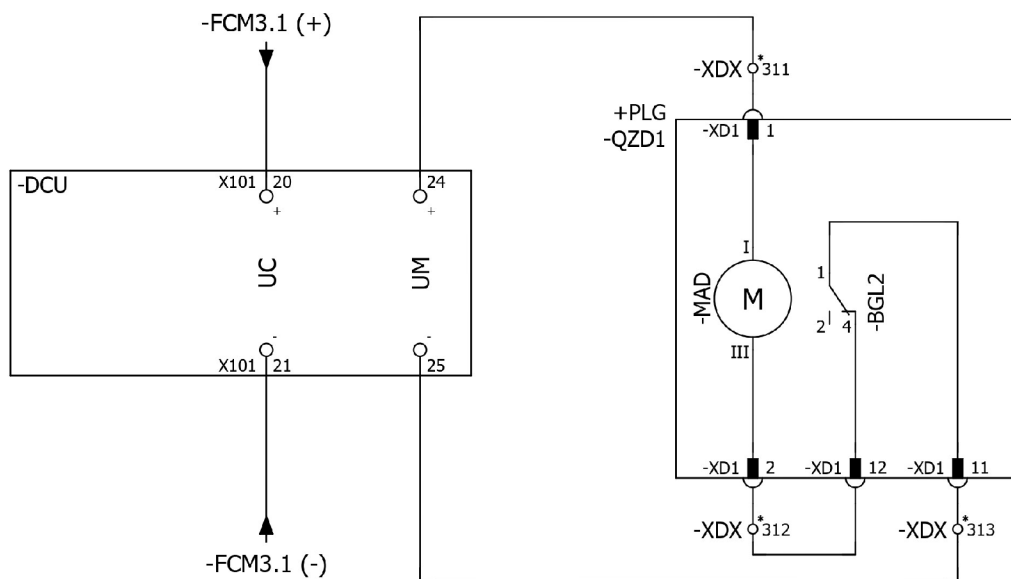
Obr. 5.7: Zjednodušené napájanie pohonu DCU
