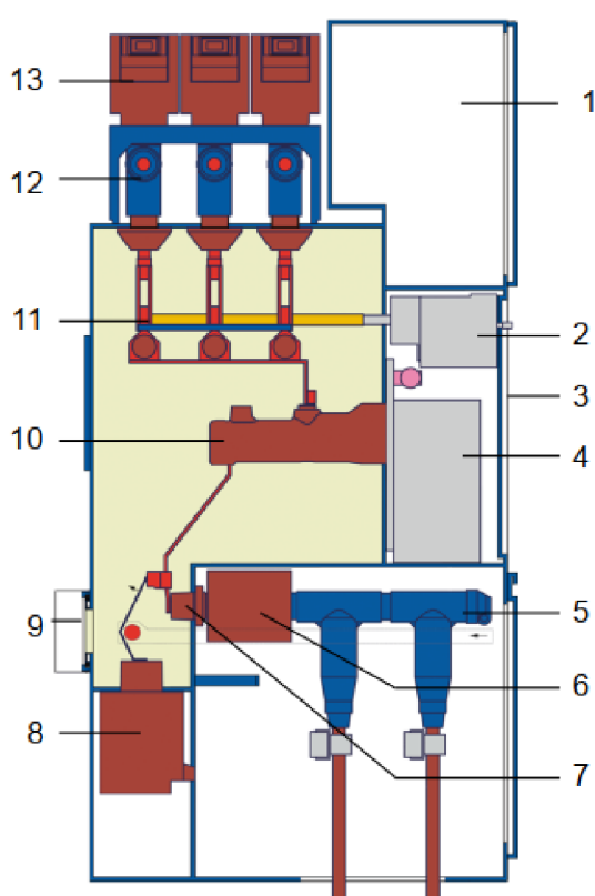
Obr. 2.1: Topológia rozvodne ZX0.2 (prevzaté zo zdroja [6])
