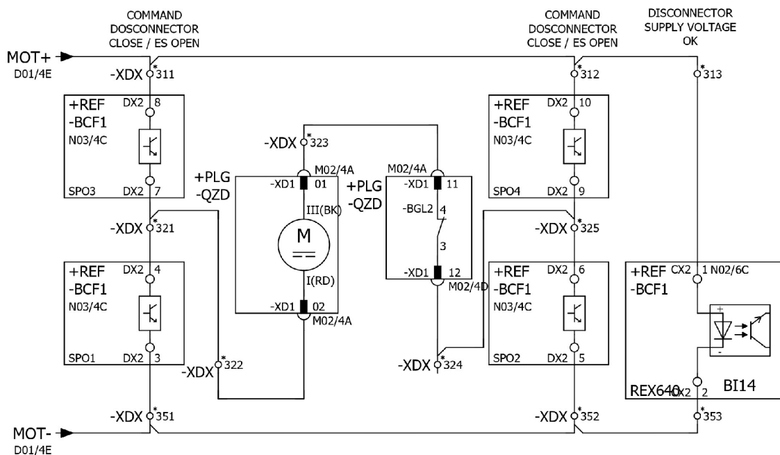
Obr. 4.2: Obvod motorového pohonu
