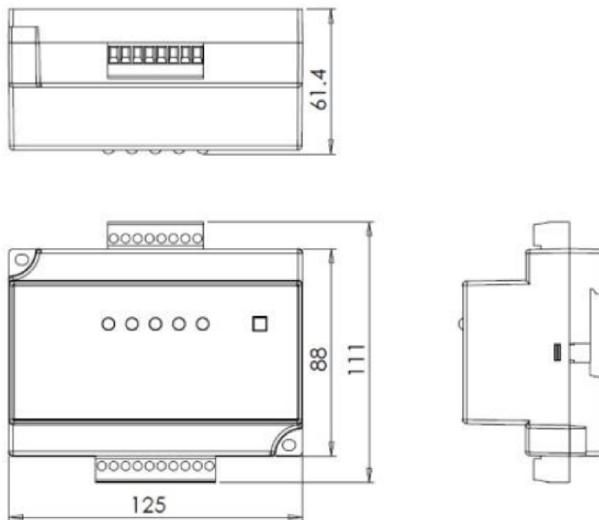
Obr. 4.6: Rozmery MCU (prevzaté zo zdroja [21])
