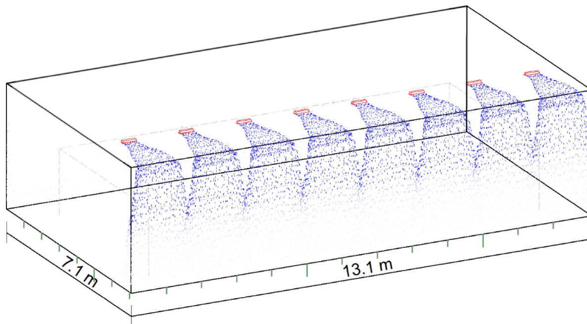
Obr. 13: Obrázek proudění vzduchu 3D - software Halton
