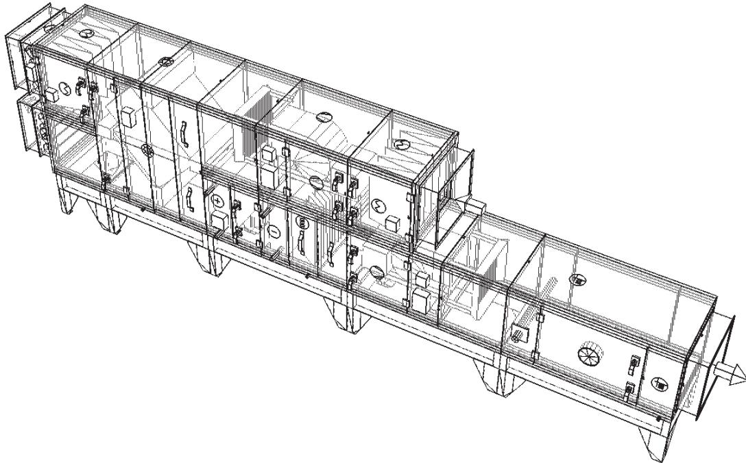
Axonometrie XYZ zezadu 02 - Zařízení 2 - Elektroléčba X = 5746 mm, Y = 750 mm, Z = 1600 mm
