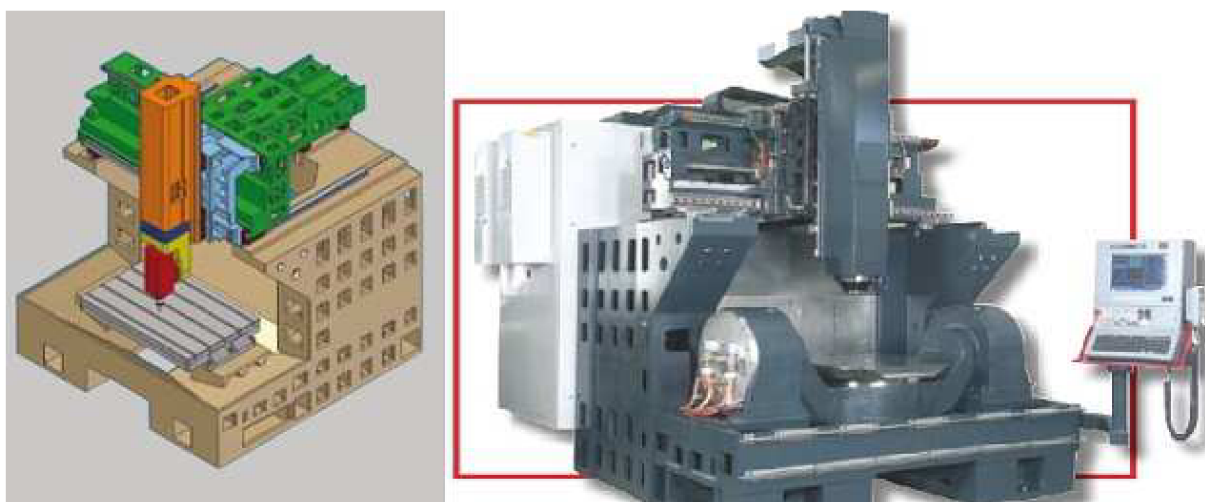
Obr. 24: G996 v provedení s pevným a otočným stolem (FIDIA) [27]
