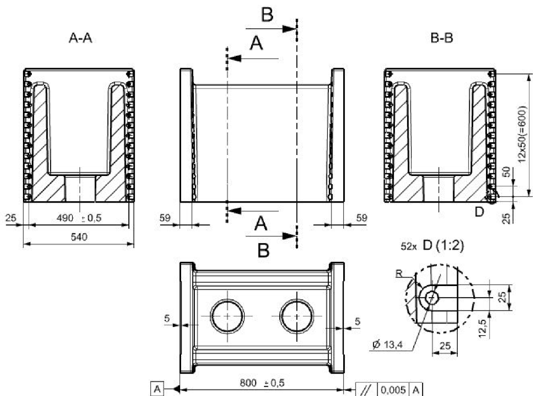
Obr. 38: Skříň připravená k sestavení s příčnicky
