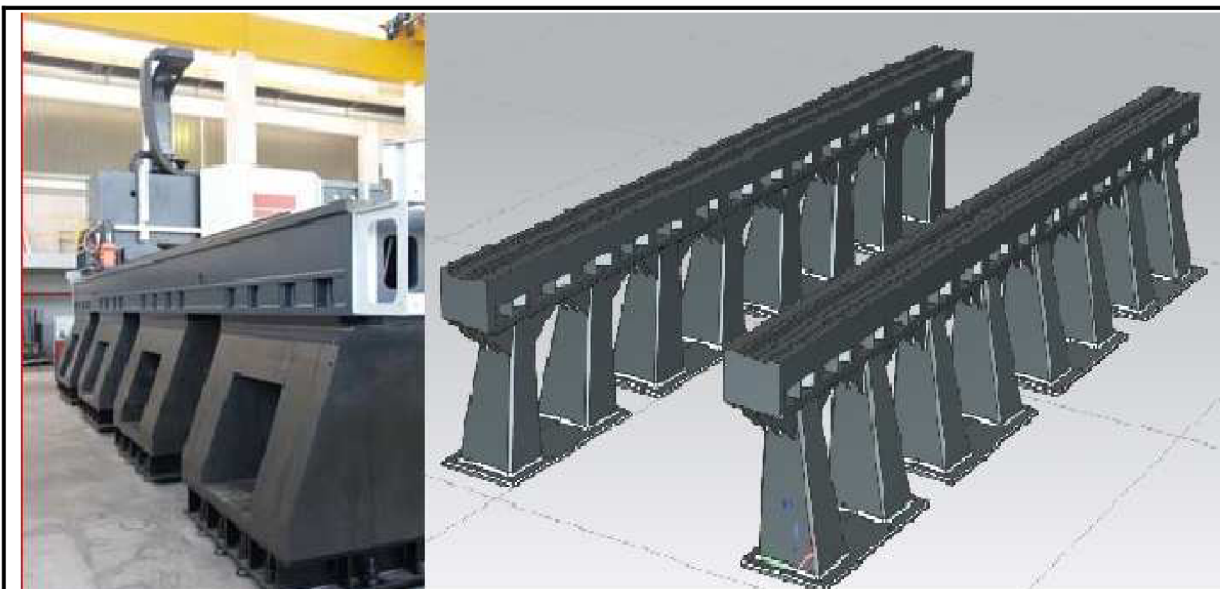
Obr. 29: Vlevo Fidia GTF, polymerbetonové stojany, nahoře litinové skříně, vpravo Náš stroj litinové stojany, litinové skříně. [27]
