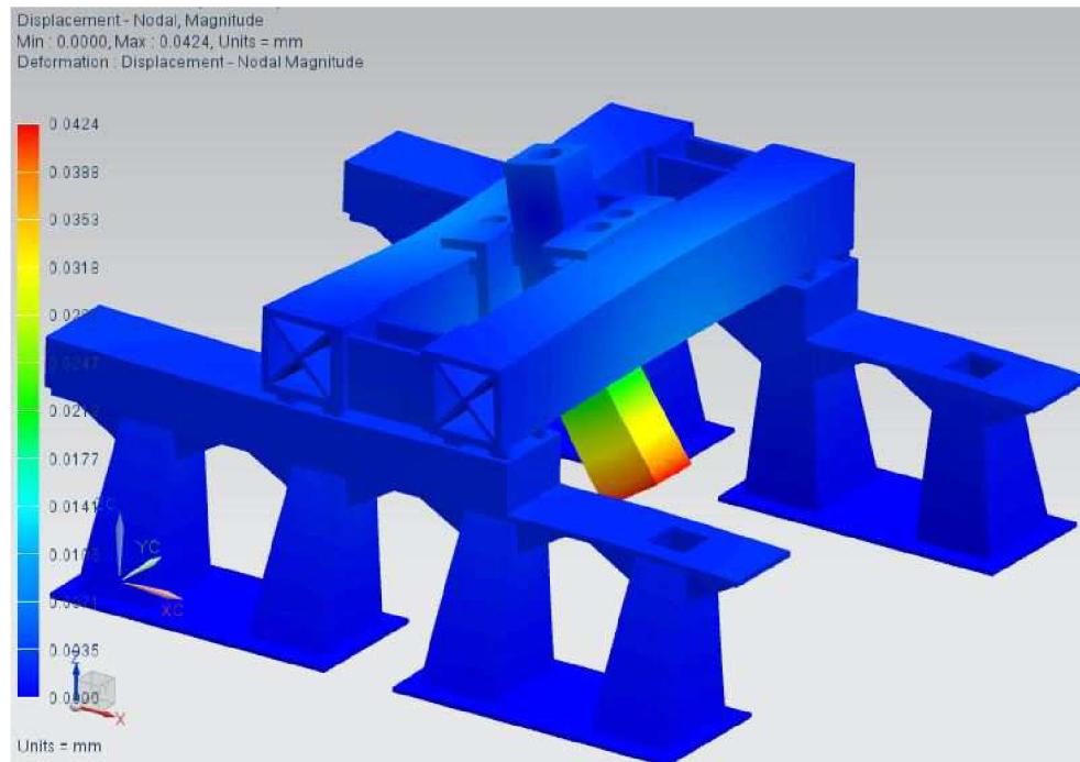
Obr. 43: Deformace stroje od obráběcí síly
