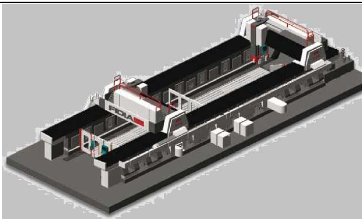
Obr. 25: GTF v provedení s dvěma příčnický (FIDIA) [27]
