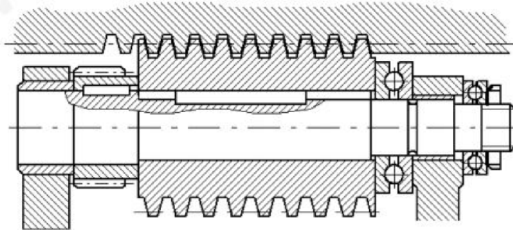
Obr. 17: Šnek a šnekový hřeben [21]
