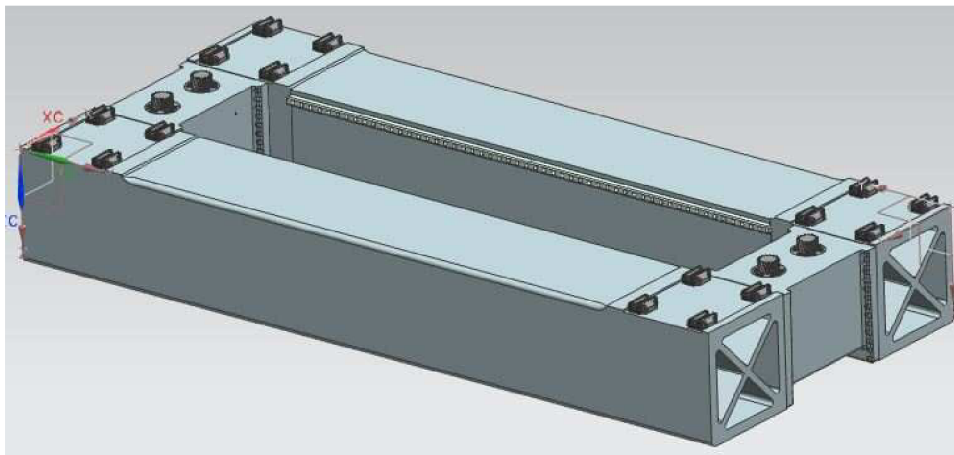
Obr. 55: Rozmístění vozíků osa X
