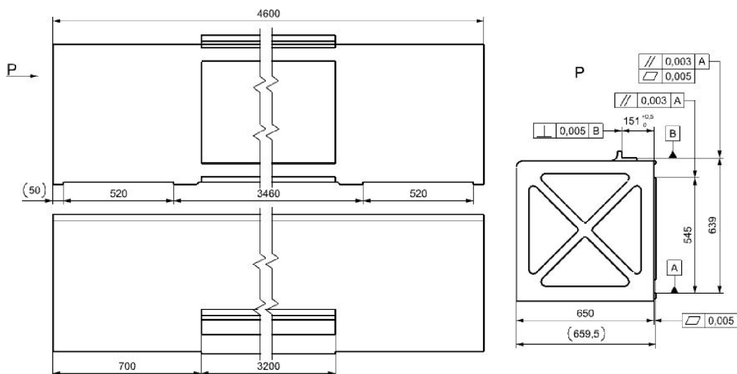
Obr. 37: Ukázka tolerancí požadovaných na sestaveném a obrobeném příčnicku
