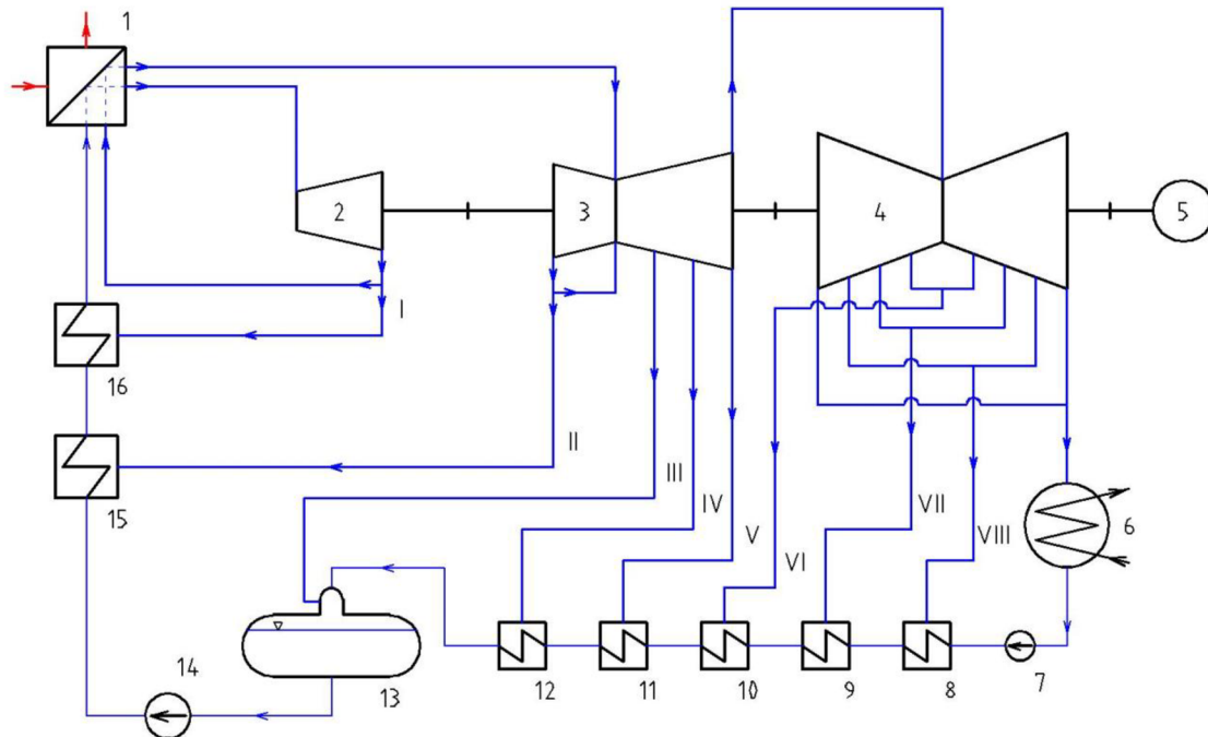
Obr. 3.1 – Zjednodušené tepelné schéma oběhu s jaderným přehříváním páry pro JE-SFR
