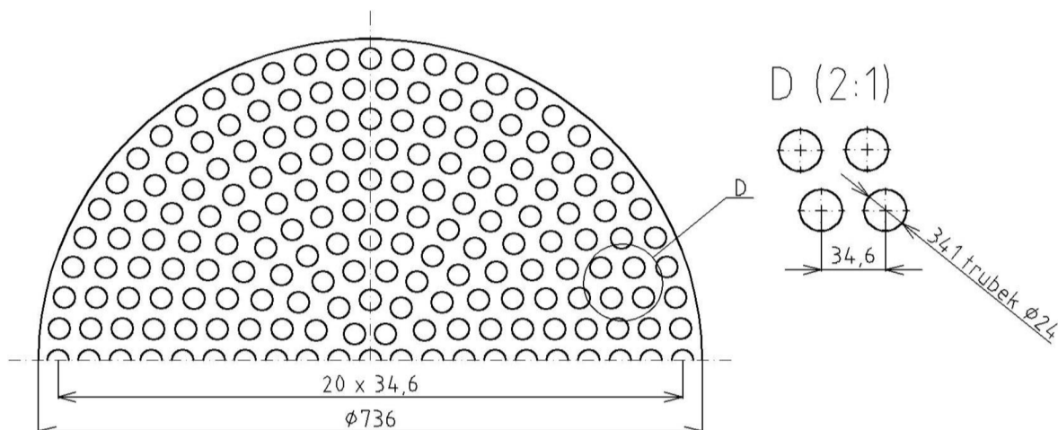
Obr. 4.4 – Schematické zobrazení řezu trubkovnicí
