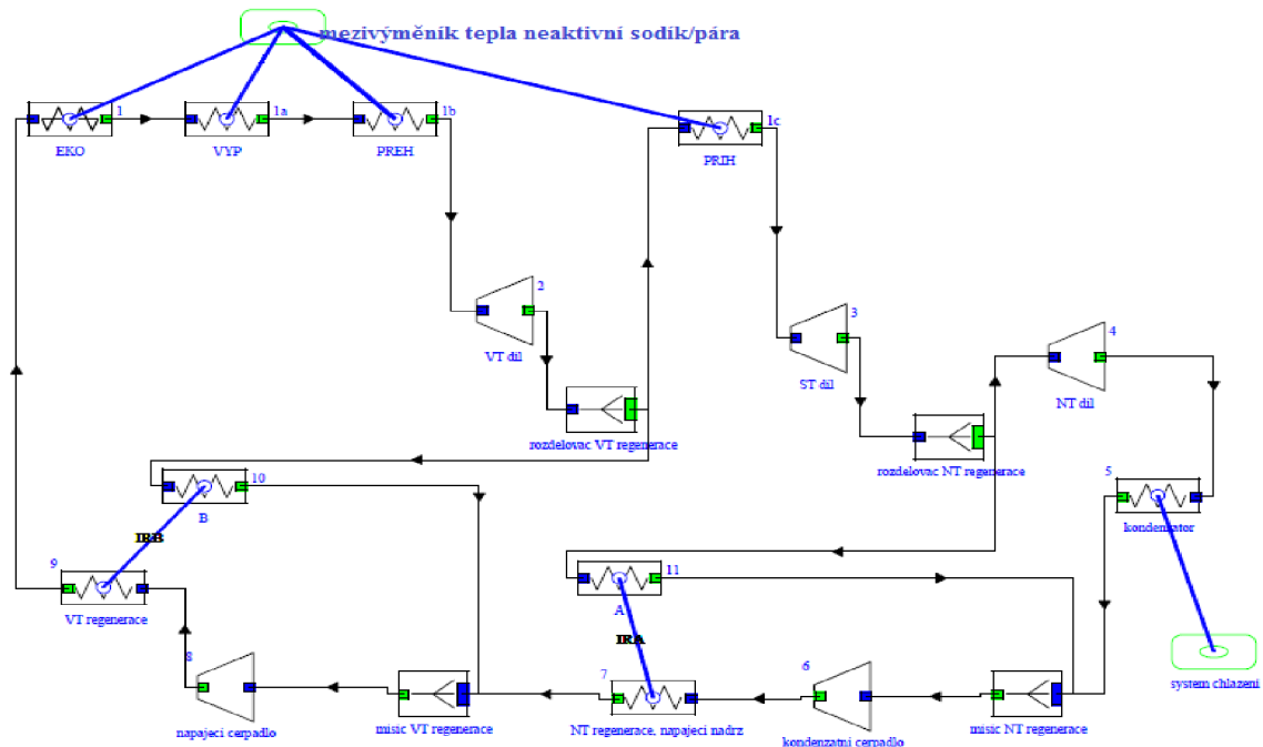
Obr. 3.2 – Znárodnění schematického zapojení systému s jaderným přehříváním páry ve školním výpočtovém programu THERMOPTIM
