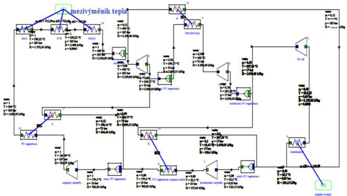
Obr. 3.7 – Znáornění schematickeho zapojení systému s nejaderným přihříváním páry včetně vypočtených hodnot ve školním výpočtovém programu THERMOPTIM
