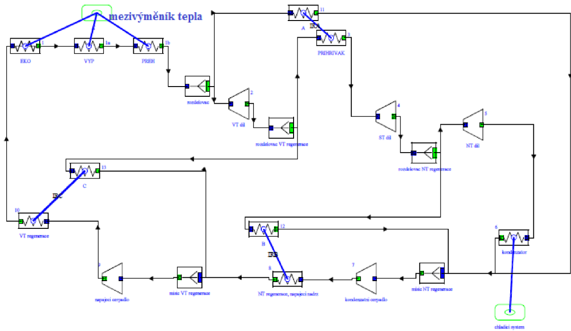
Obr. 3.6 – Znáornění schematickeho zapojení systému s nejaderným přihříváním páry ve školním výukovém programu THERMOPTIM
