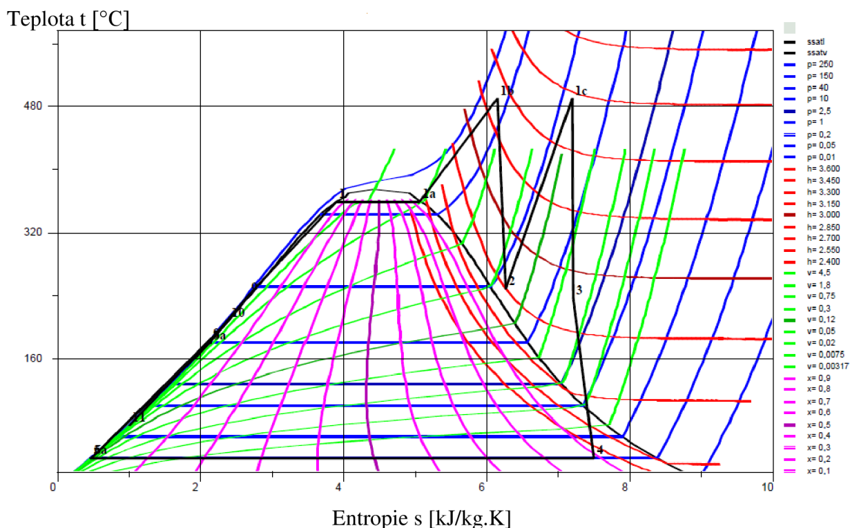
Obr. 3.4 – Znáznornění systému s jaderným přehříváním páry v T-s diagramu
