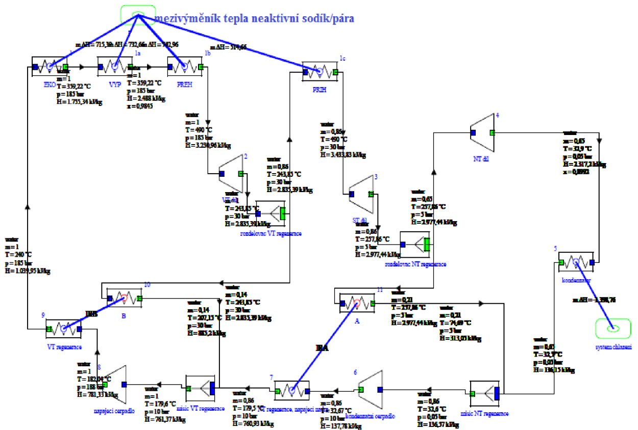
Obr. 3.3 – Znárodnění schematického zapojení systému s jaderným přehříváním páry včetně vy-početných hodnot ve školním výpočtovém programu THERMOPTIM
