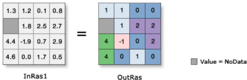
Obrázek 14: Vizuální zobrazení nástroje Int
