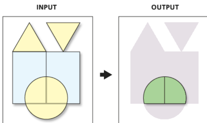
Obrázek 18: Vizuální zobrazení nástroje Intersect na příkladu polygonů
