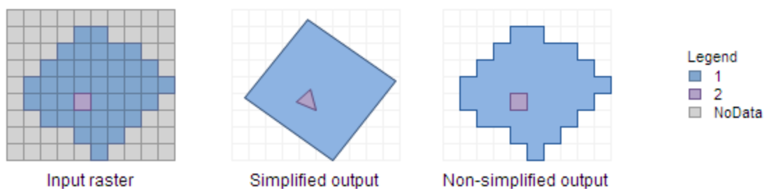
Obrázek 15: Vizuální zobrazení nástroje Raster to Polygon
