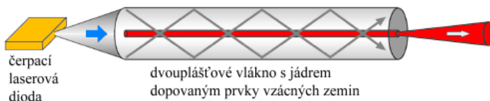
Obr. 20 Schéma vláknového laseru [48]
