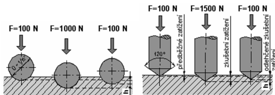
Obr. 36 Metoda měření tvrdosti podle Rockwella [28]
