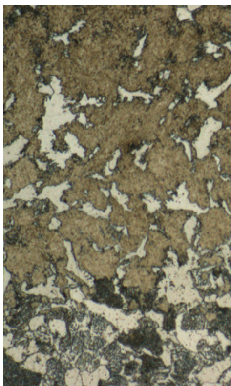
Obr. 66 Detail C - Přechod TOO a ZM, zvětšení 1200x
