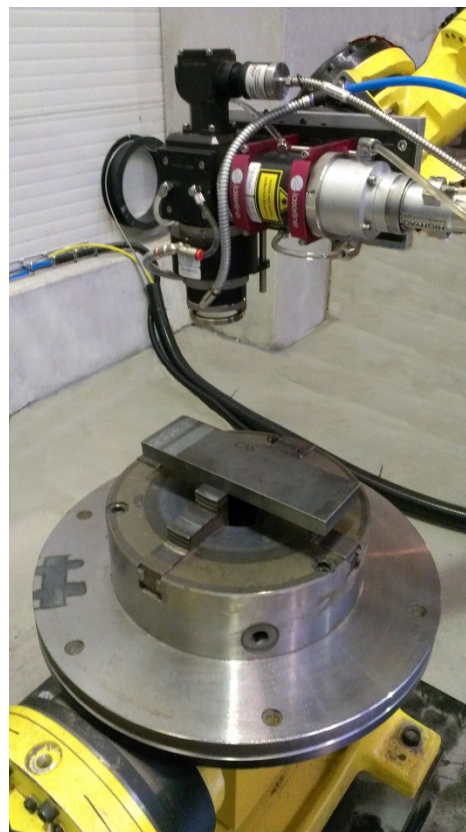
Obr. 39 Laserové pracoviště
