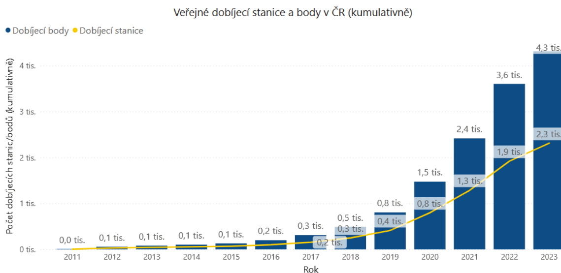
Obr. 14 – Vývoj počtu veřejných dobíjecích stanic a bodů v ČR v letech 2011-2023 | zdroj [60]
