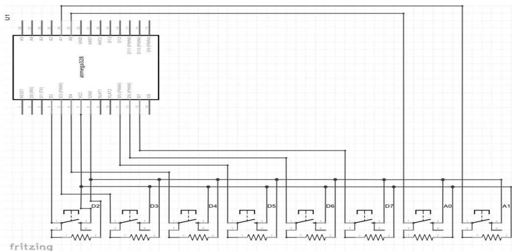
Obr.10: Princíp zapojenie ovládacích prvkov v programe Fritzing
