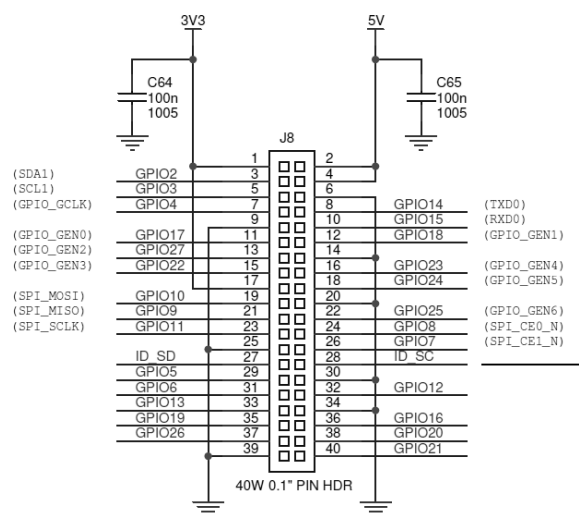
Obr. 4: Raspberry Pi B+ vstup/výstupy [8]
