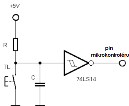
Obr. 11: Bezzákmitové tlačidlo [17]
