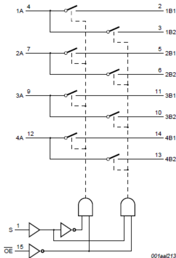
Obr. 12: Funkčný diagram 74CBTLV3257 [20]
