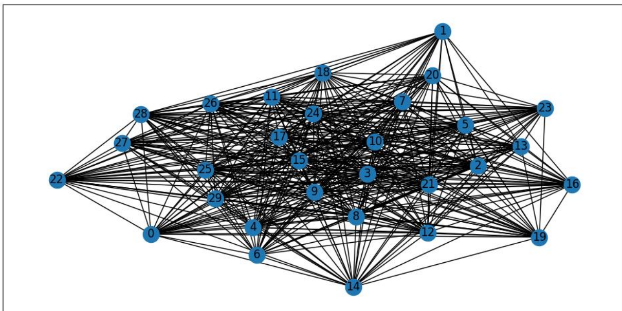
Obrázek 5.8 Graf podobností
