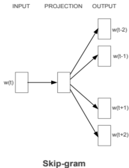
Obrázek 3.3 Skip-gram architektura [6]
