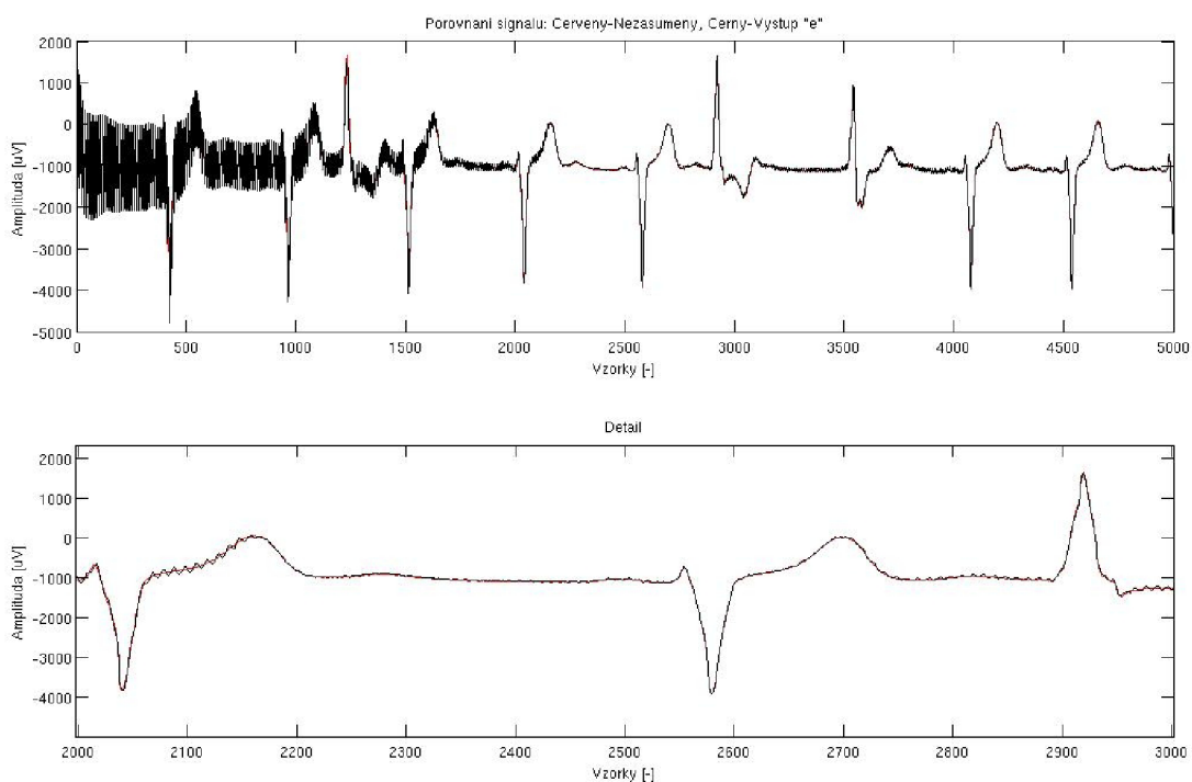
Obr. 2.19: Vyfiltrovaný signál při použití brumového schématu a algoritmu signum signum - první signál. Tab 2.9
