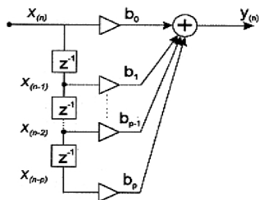
Obr. 1.3: Model klouzavých součtů.
