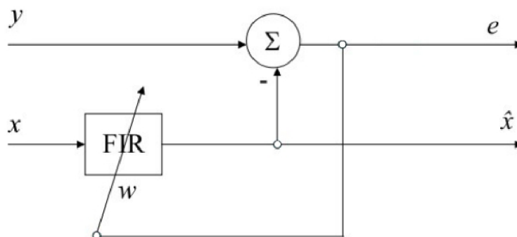
Obr. 1.5: Základní schéma adaptace.
