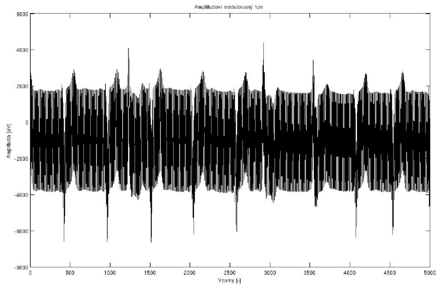
Obr. 2.2: Zašumněný signál.
