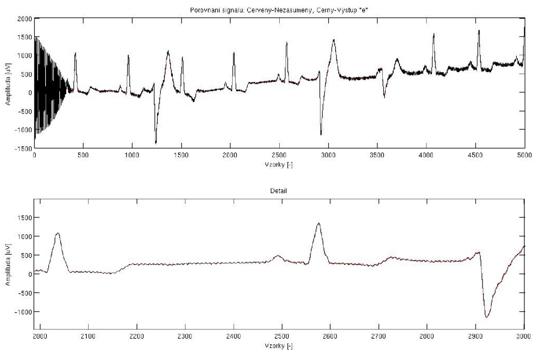
Obr. 2.20: Vyfiltrovaný signál při použití brumového schématu a algoritmu signum signum - druhý signál. Tab 2.9
