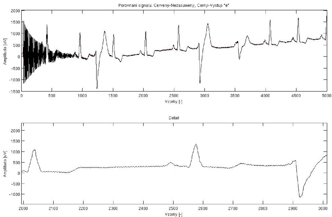
Obr. 2.15: Vyfiltrovaný signál při použití brumového schématu a obecného adaptačního algoritmu - druhý signál. Tab 2.6
