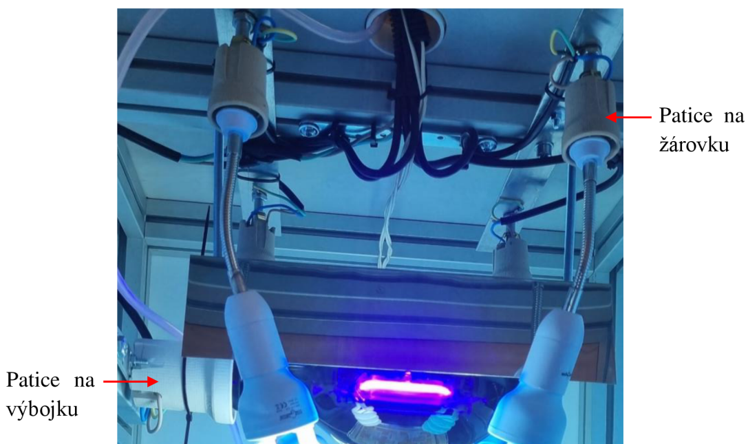
Obrázek 15: Upevnění rtuťové výbojky UV black light 400 W a žárovek Repti Planet UVB 26 W pomocí patic.
