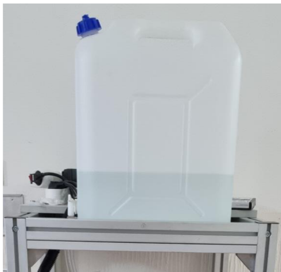
Obrázek 12: Nádoba na kapalinu v přístroji na simulaci degradace materiálů (PSDM).
