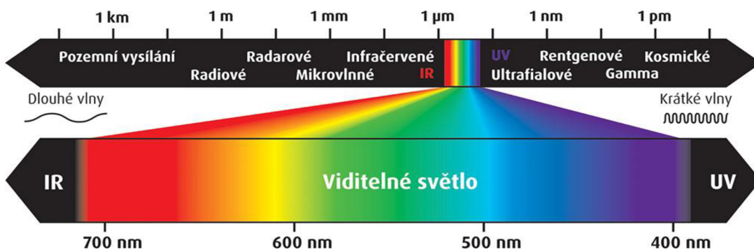
Obrázek 2: Elektromagnetické spektrum [24].
