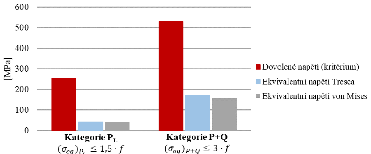
Obr. 39 Přechodový díl – vyhodnocení napětí
