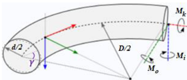
Obr. 10 Oblouky – přídavné momenty [15]
