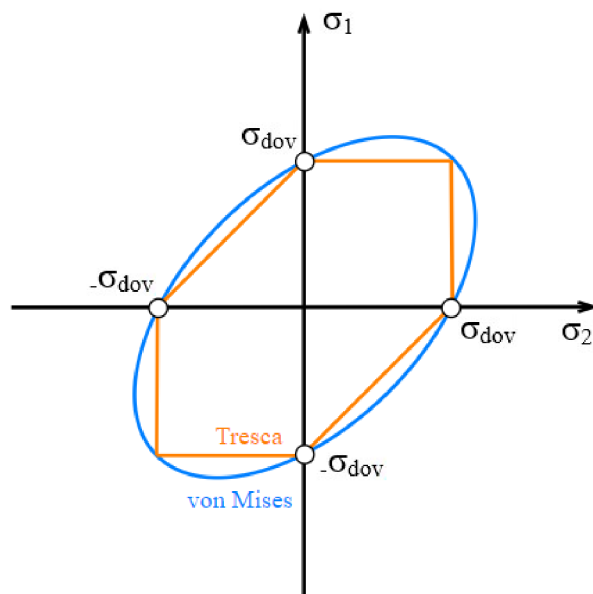
Obr. 6 Teorie porušení – Tresca a von Mises (dvouosá napjatost)
