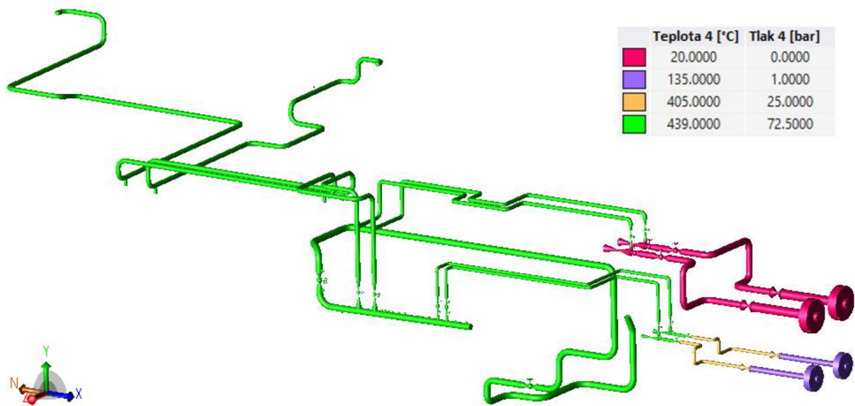
Obr. 23 3D model – procesní parametry pro provozní stav 3
