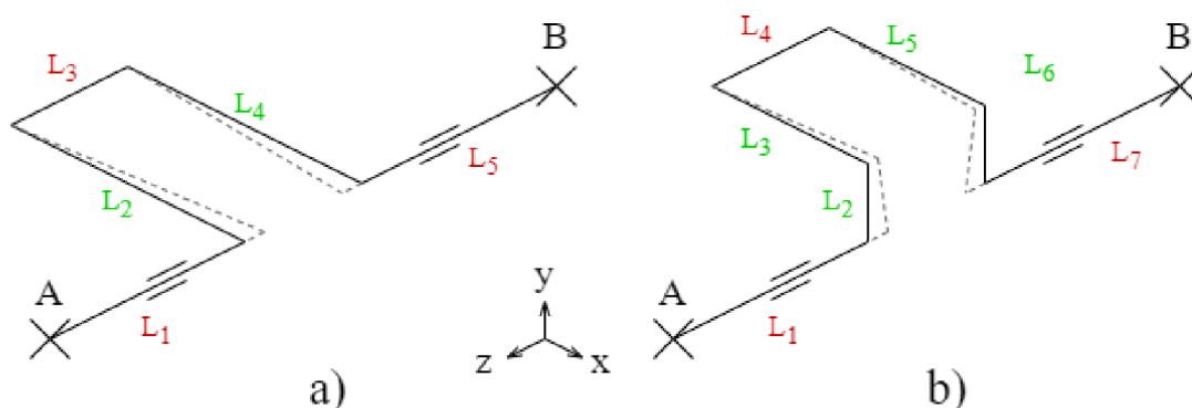
Obr. 17 Tvarový kompenzátoz – a) 2D smyčka (U-kompensátor), b) 3D smyčka
