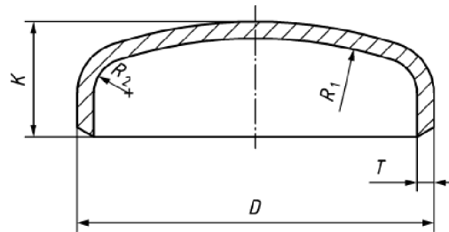
Obr. 14 Tlakové dno [13]
