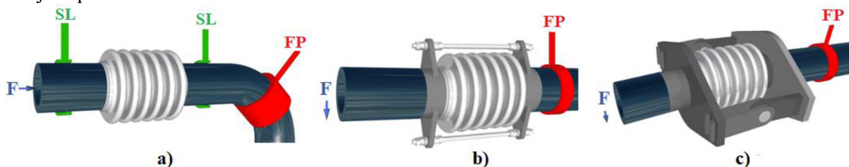
Obr. 18 Vlnovcový kompenzátoz – a) axiální, b) laterální, c) angulární [20]
