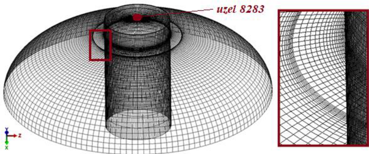
Obr. 38 Přechodový díl – výpočtová síť (PRG NozzlePRO)
