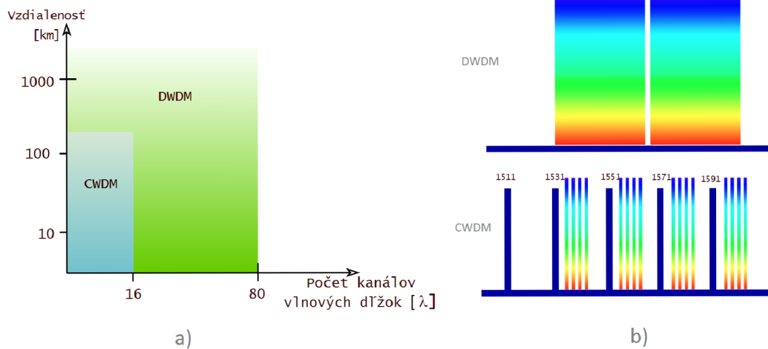
Obr. 3.3: a) Približný počet kanálov v DWDM s naznačeným dosahom oproti CWDM b) Náhľad na rozdiely medzi DWDM a CWDM z hľadiska hustoty vlnových dĺžok. [32]
