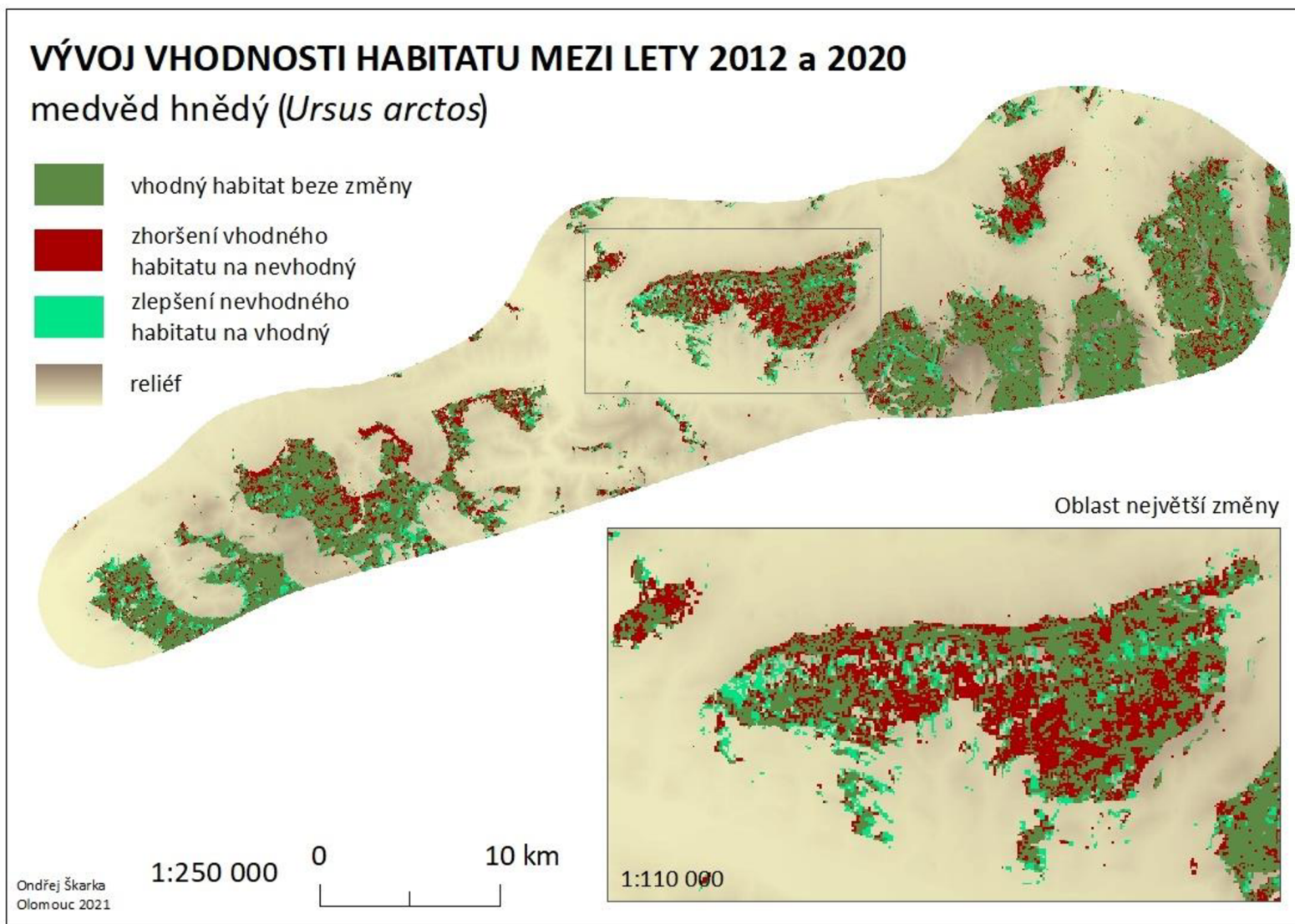
Mapa 7. Vývoj vhodnosti habitatu medvěda hnědého ( Ursus arctos ) mezi lety 2012 a 2020.
