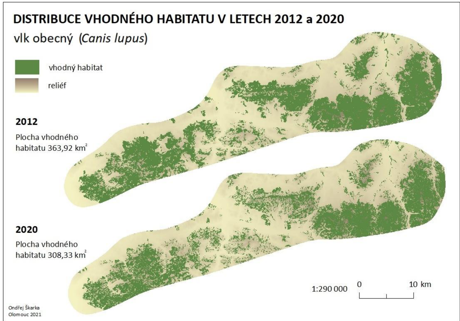
Mapa 4. Habitatové modely pro vlka obecného ( Canis lupus ).
