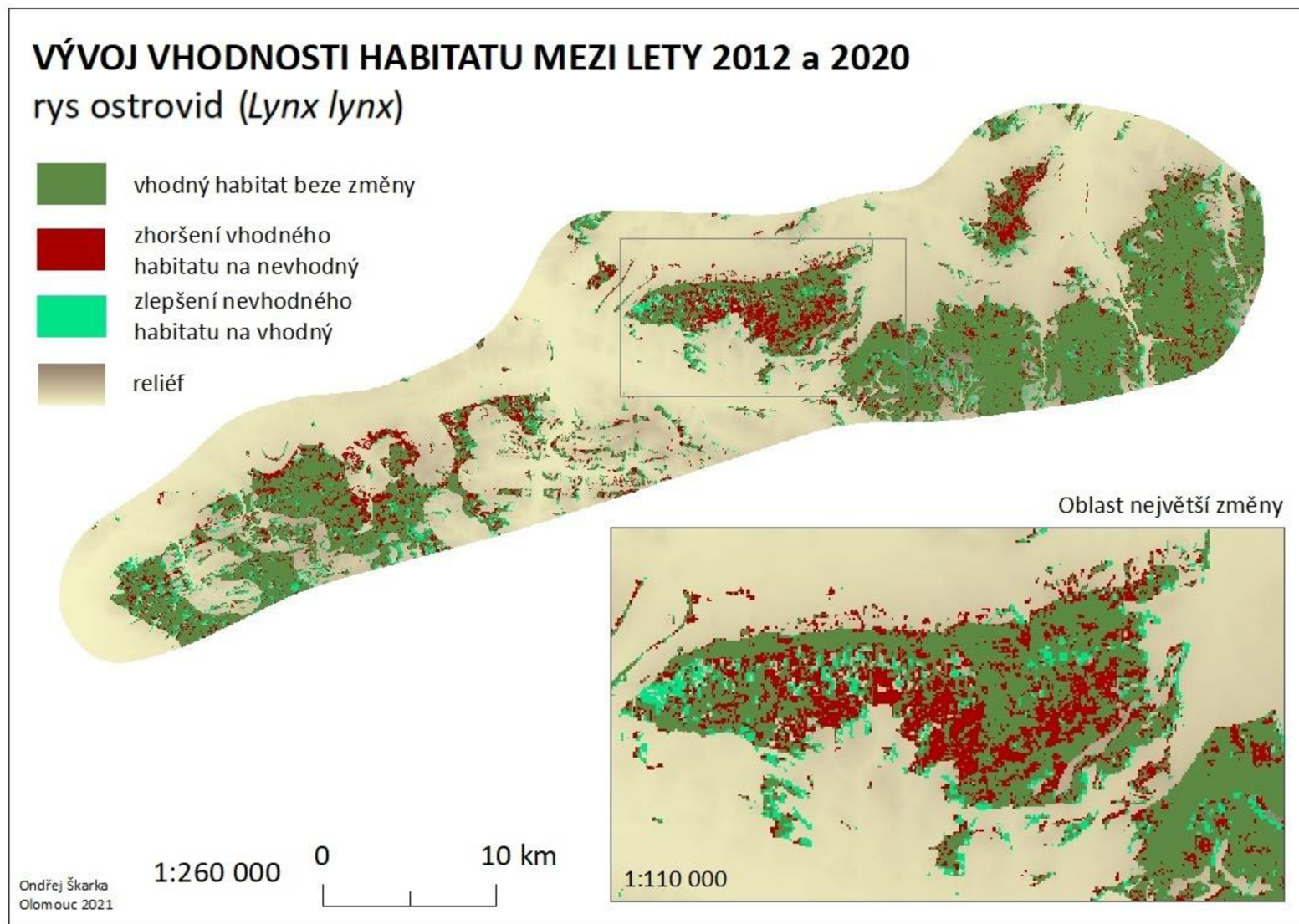
Mapa 3. Vývoj vhodnosti habitatu rysa ostrovida ( Lynx lynx ) mezi lety 2012 a 2020.
