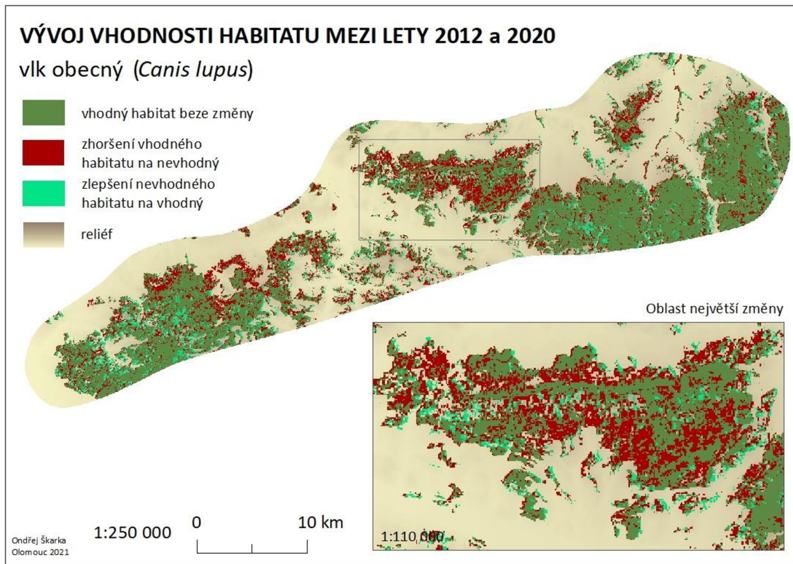
Mapa 5. Vývoj vhodnosti habitatu vlka obecného ( Canis lupus ) mezi lety 2012 a 2020.
