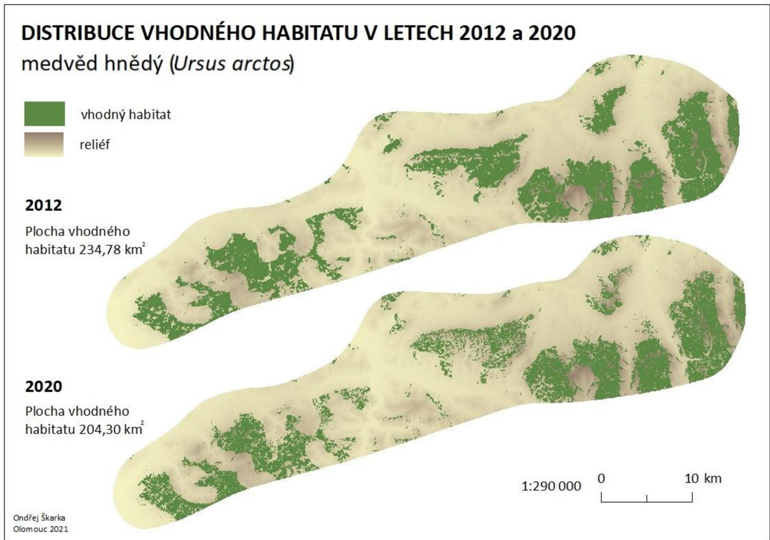
Mapa 6. Habitatové modely pro medvěda hnědého ( Ursus arctos ).
