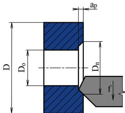
Obr. 17 Princip čelní krátkodobé zkoušky [8].
