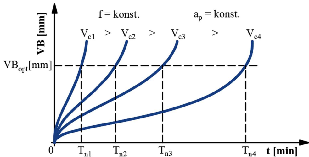
Obr. 14 Křivky otupení [8].
