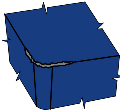
Obr. 9 Vyštipování ostří [30].
