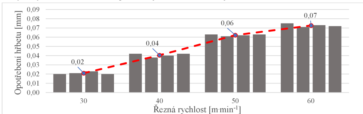
Obr. 50 Opatřebení nástroje pro ADIT vzorek.
