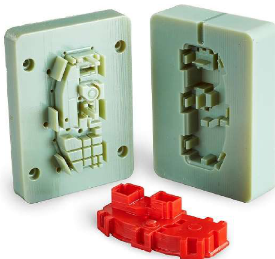
Obr. 19 Forma vyrobená aditivní technologií PolyJet [42].
