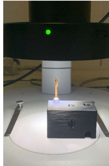
b) upevnění nástroje v přípravku
