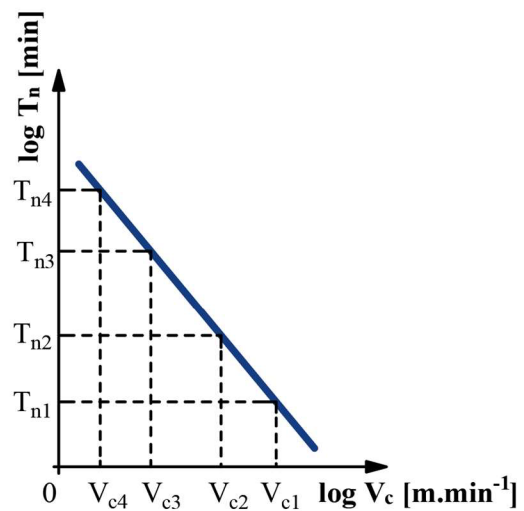
Obr. 16 Závislost trvanlivosti na řezné rychlosti [8].
