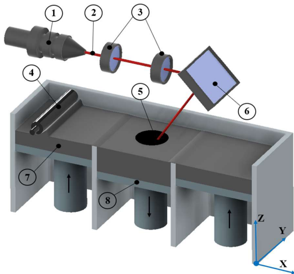
Obr. 26 Princip metody SLM [65].
