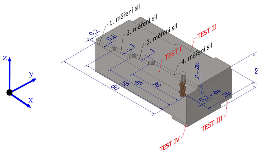
Obr. 30 Metodika testování.
