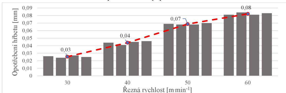
Obr. 51 Opatřebení nástroje pro ADIT-TZ vzorek.
