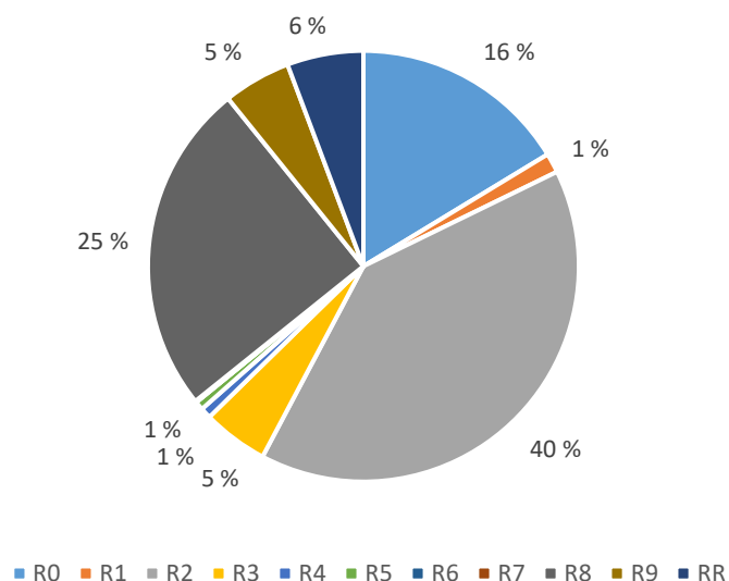
Graf č. 26 Obsahová analýza L&L
