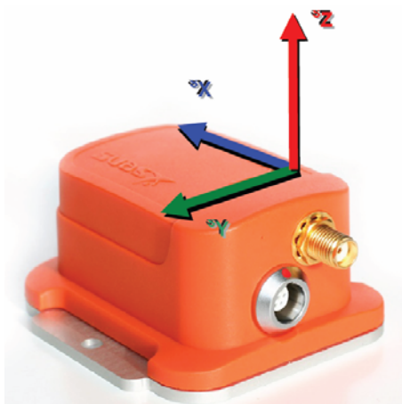
Obr. 2.2: Súradnicový systém snímača viazaný na puzdro MTi-G [1]
