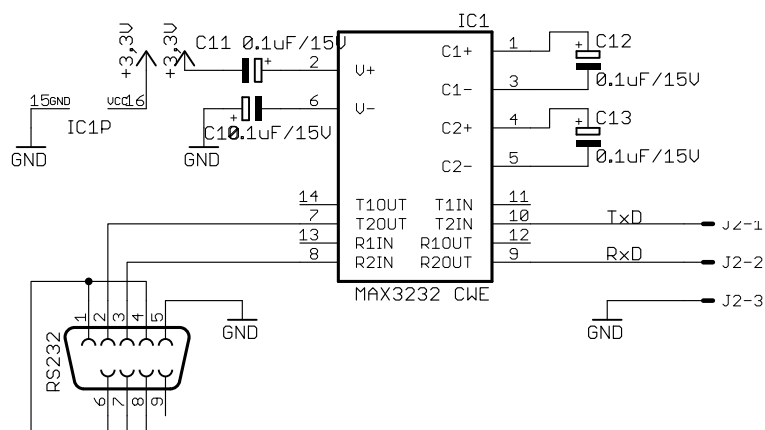
Obr. 5.1: Zapojenie obvodu MAX 3232
