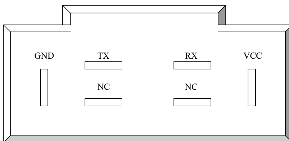
Obr. 5.5: Konektor snímača MTi-G na strane prevodníku RS 232
