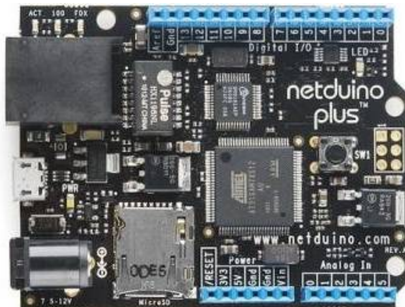
Obr. 3.1: Netduino Plus
