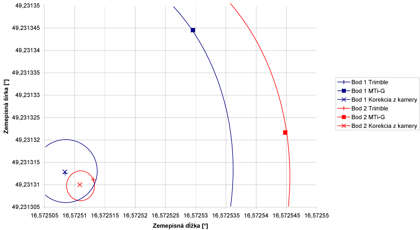
Meranie polohy v okolí značky číslo 3 v systéme ETRS
