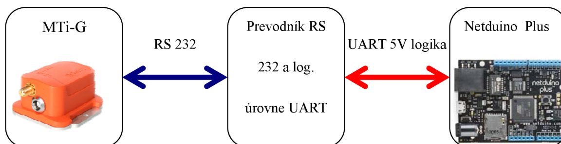
Obr. 5.4: Prepojenie Netduino a MTi-G
