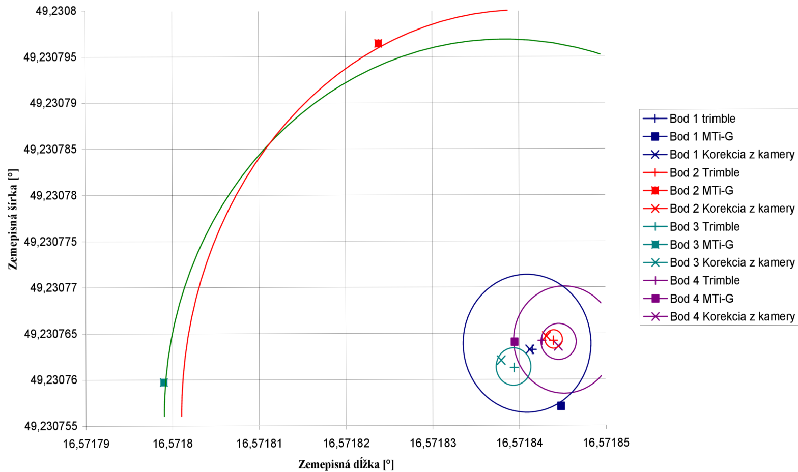
Meranie polohy v okolí značky číslo 6 v systéme ETRS
