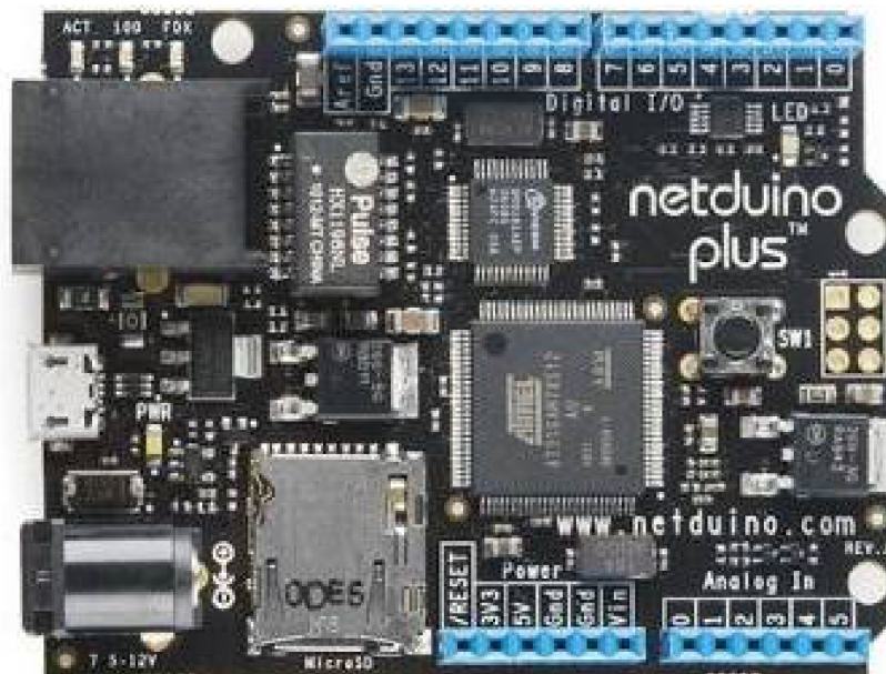
Obr. 3.1: Netduino Plus
