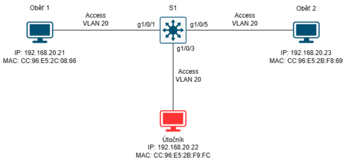
Obr. 31 Topologie sítě při útoku ARP spoofing.
