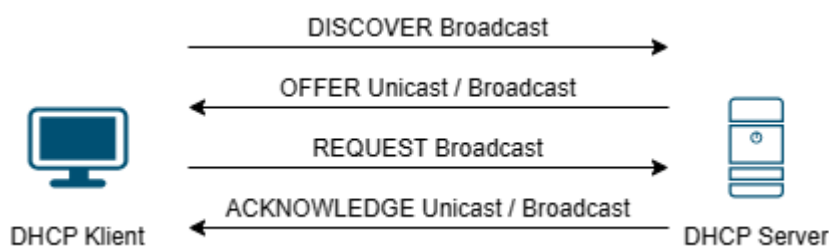
Obr. 17 Proces komunikace DHCP.
