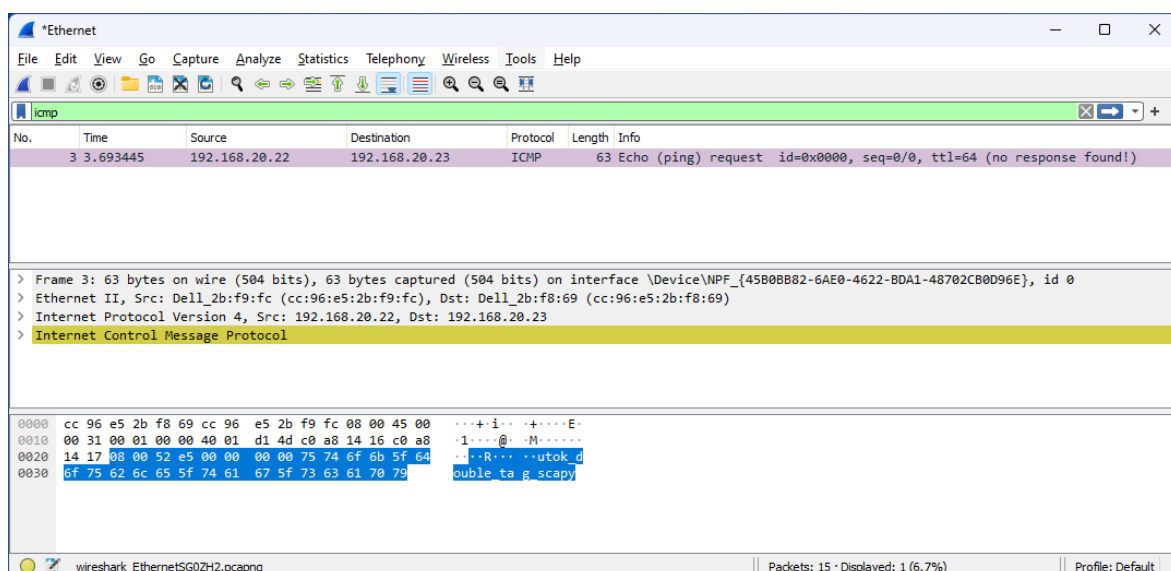
Obr. 30 Zachycení podvržené ICMP zprávy na PC oběti (double tagging).
