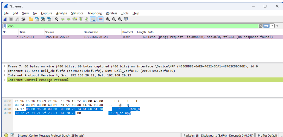
Obr. 28 Zachycení podvržené ICMP zprávy na PC oběti (switch spoofing).
