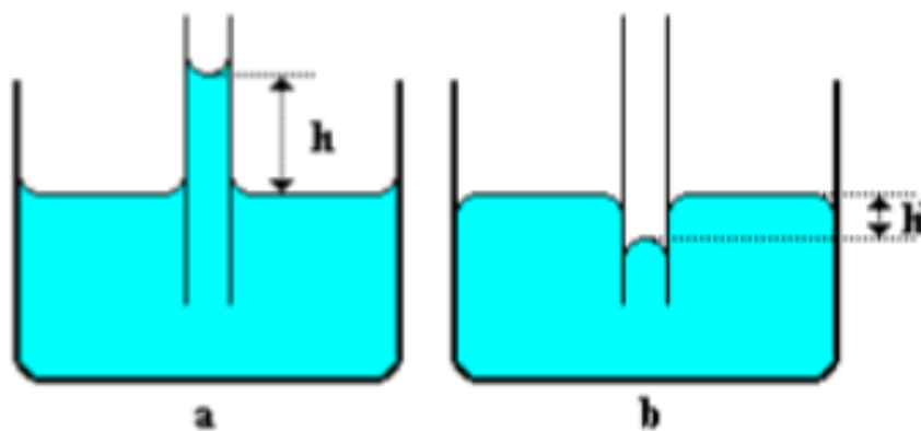
Obrázek 11: Kapilární jevy
