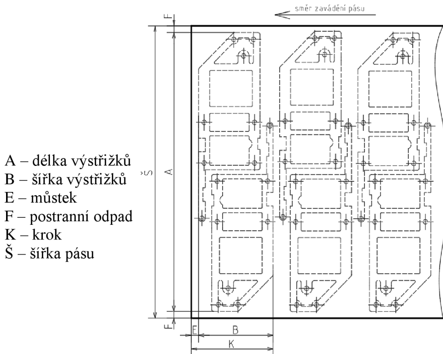
obr. 36 Uspořádání č.3
