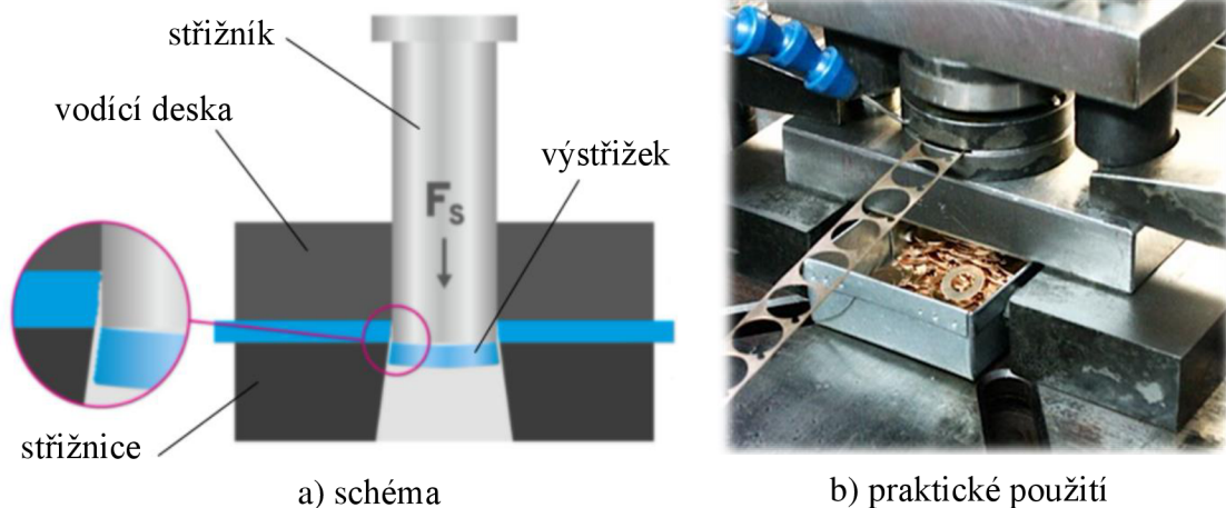
Obr. 8 Stříhání [17; 18].
