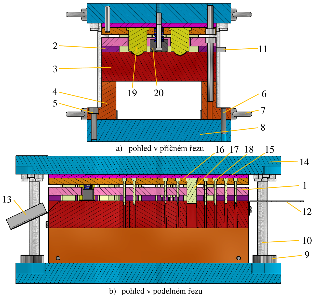
Obr. 44 Sdružený nástroj.
