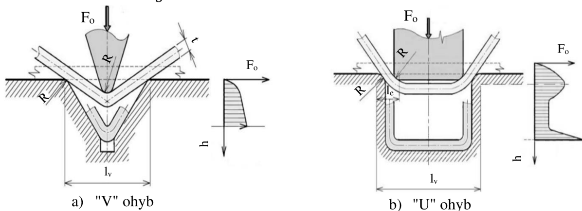
Obr. 24 Typy ohýbání [3].
