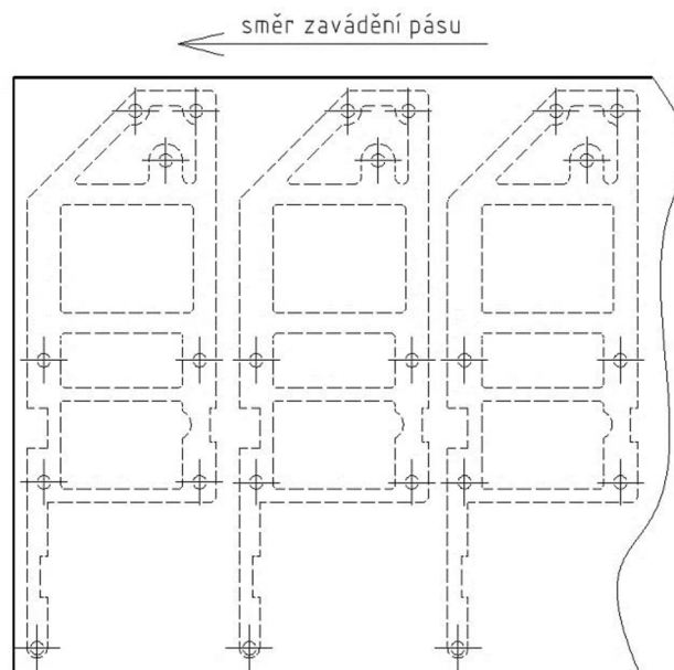
obr. 35 Uspořádání č.2
