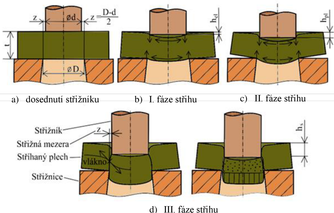
Obr. 10 Průběh stříhání [3].
