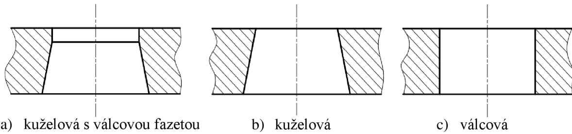
Obr. 19 Vnitřní tvary střížnic [20].
