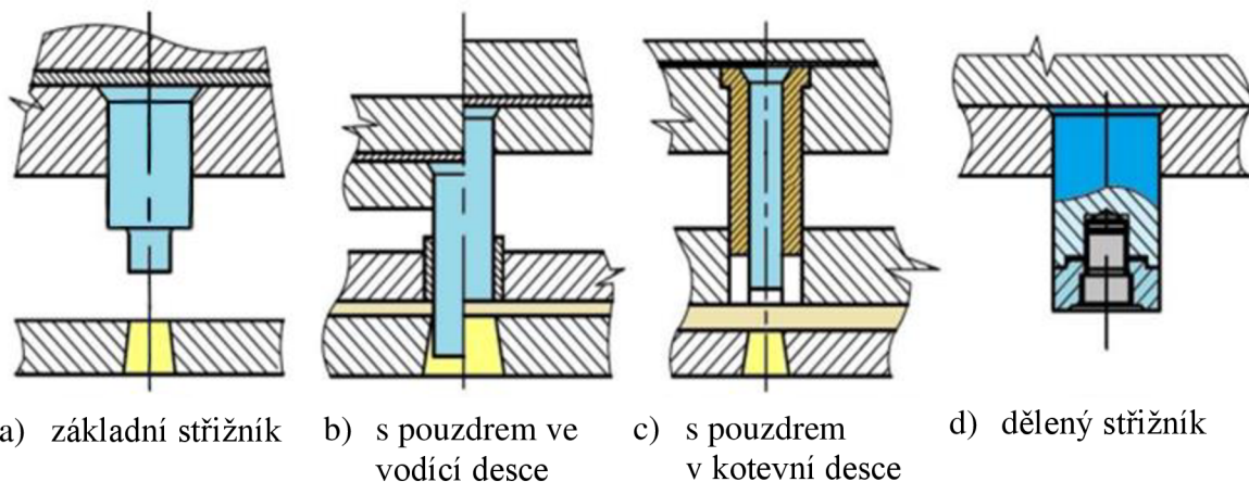
Obr. 18 Konstrukce střížníků [20].
