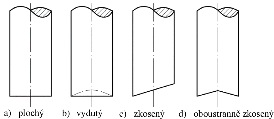
Obr. 17 Tvary střížníků [19].
