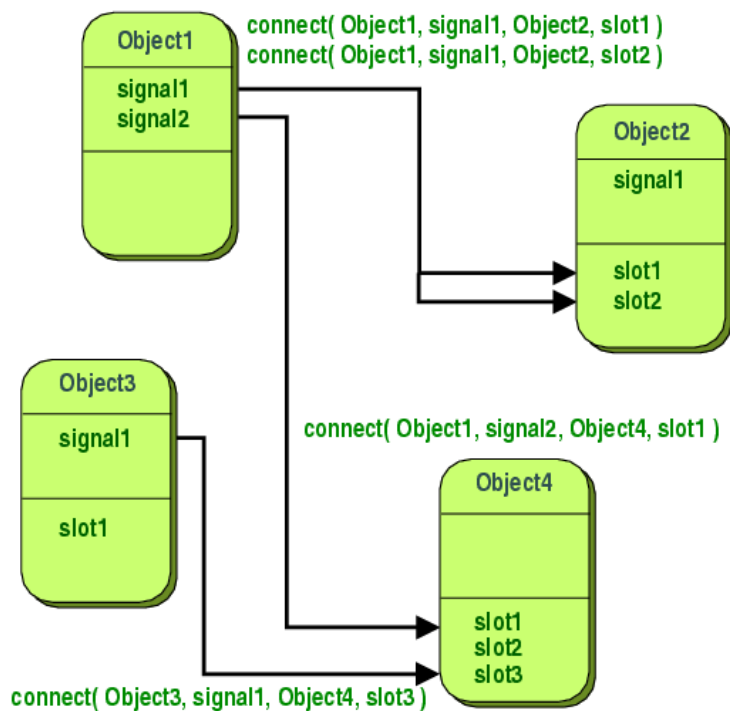
Obrázek 3.1 Signály a sloty v Qt
