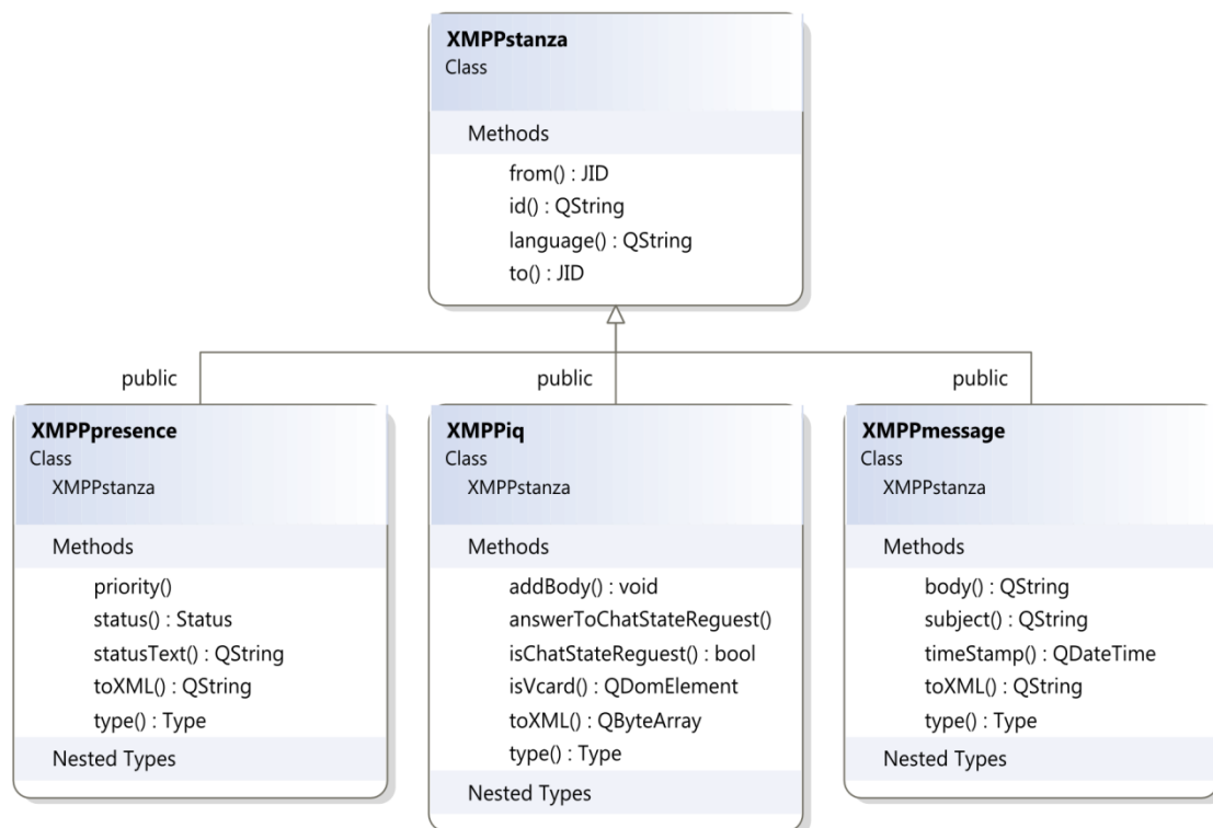
Obrázek 6.4 Třídy reprezentující jednotlivé XMPP stanzy
