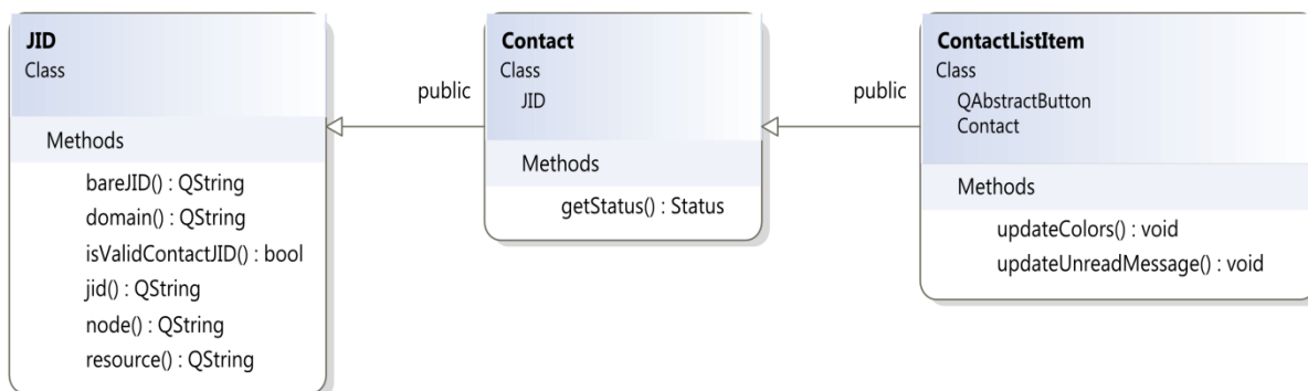
Obrázek 6.3 Hierarchie dědičnosti třídy ContactListItem
