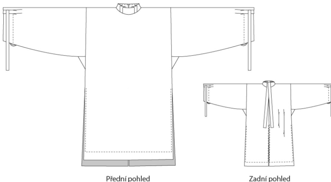
Obr. 95: Technický náčrt košile
