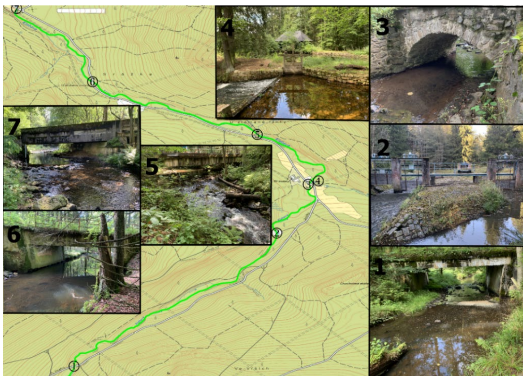
Obrázek 8 – technické objekty na spodní části hodnoceného úseku: 1 – Most Josefka, 2 – vzdouvací stavba se stavidlem, 3 – propustek pod silnicí, 4 – vodní elektrárna, 5 – most u zlámané lávky, 6 – most U druhého mostu, 7 most u Strašic (zdroj: vlastní)
