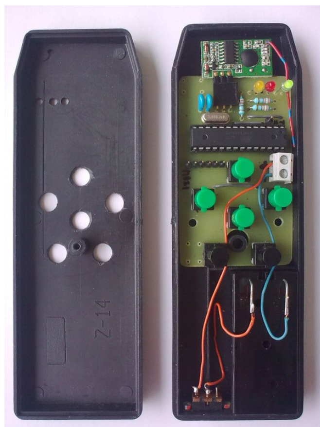
Obrázek C.3: Elektronika ovladače
