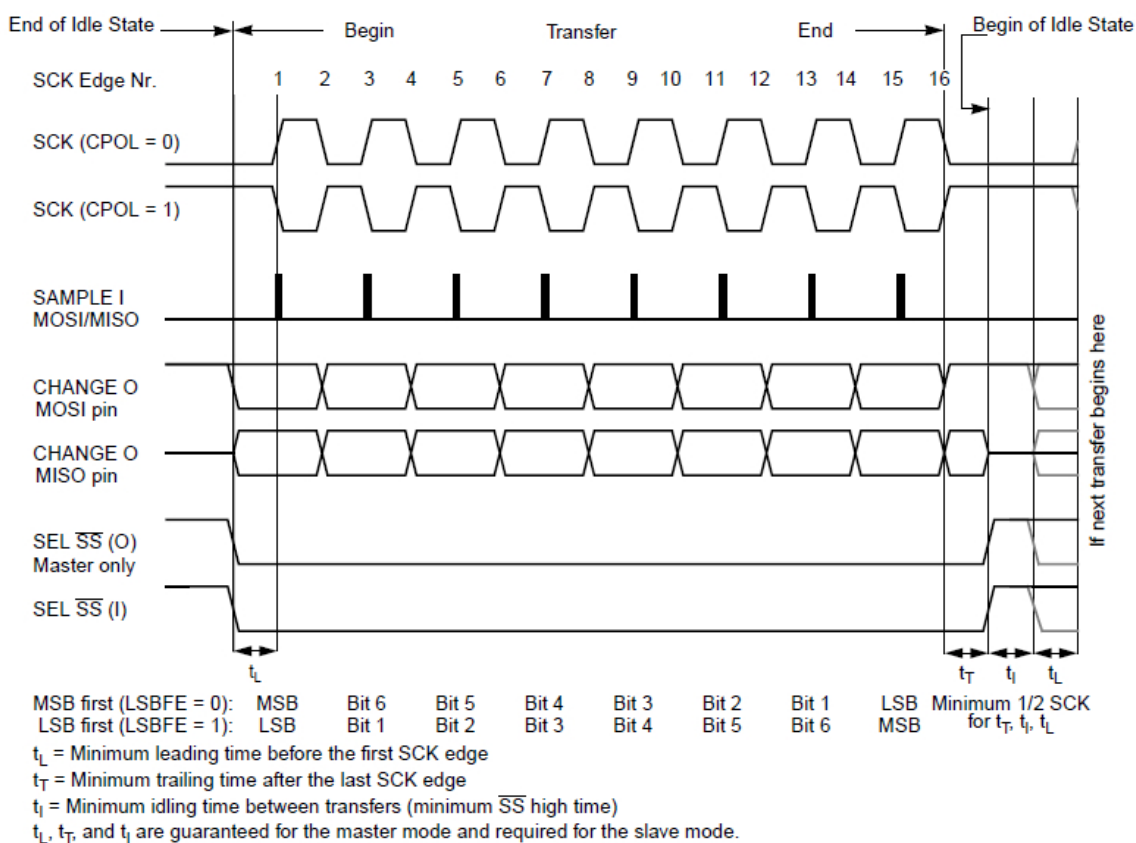
Obrázek 2.2: Časové průběhy rozhraní SPI při CPHA=0
